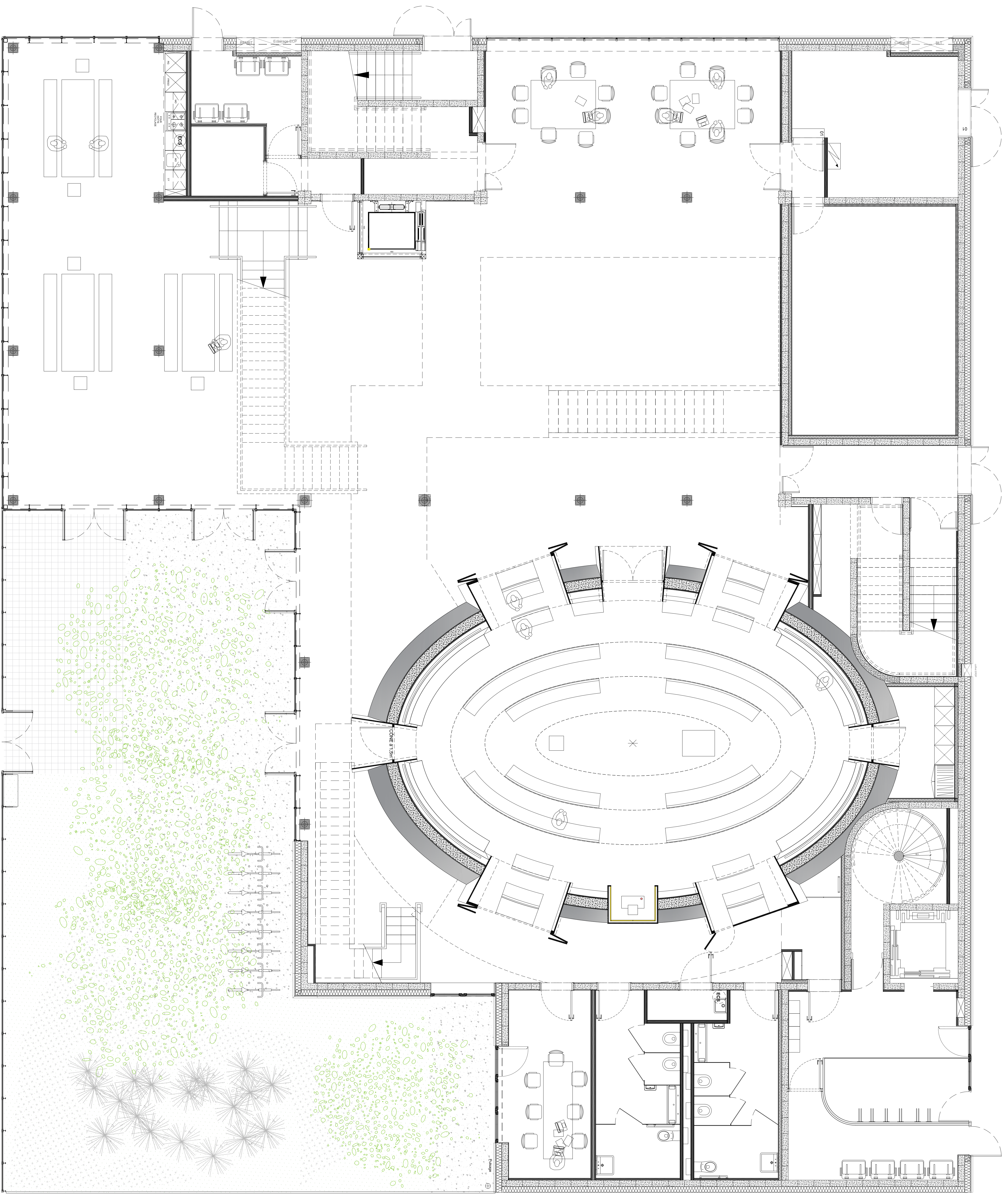
Plan du Rez-de-chaussée
