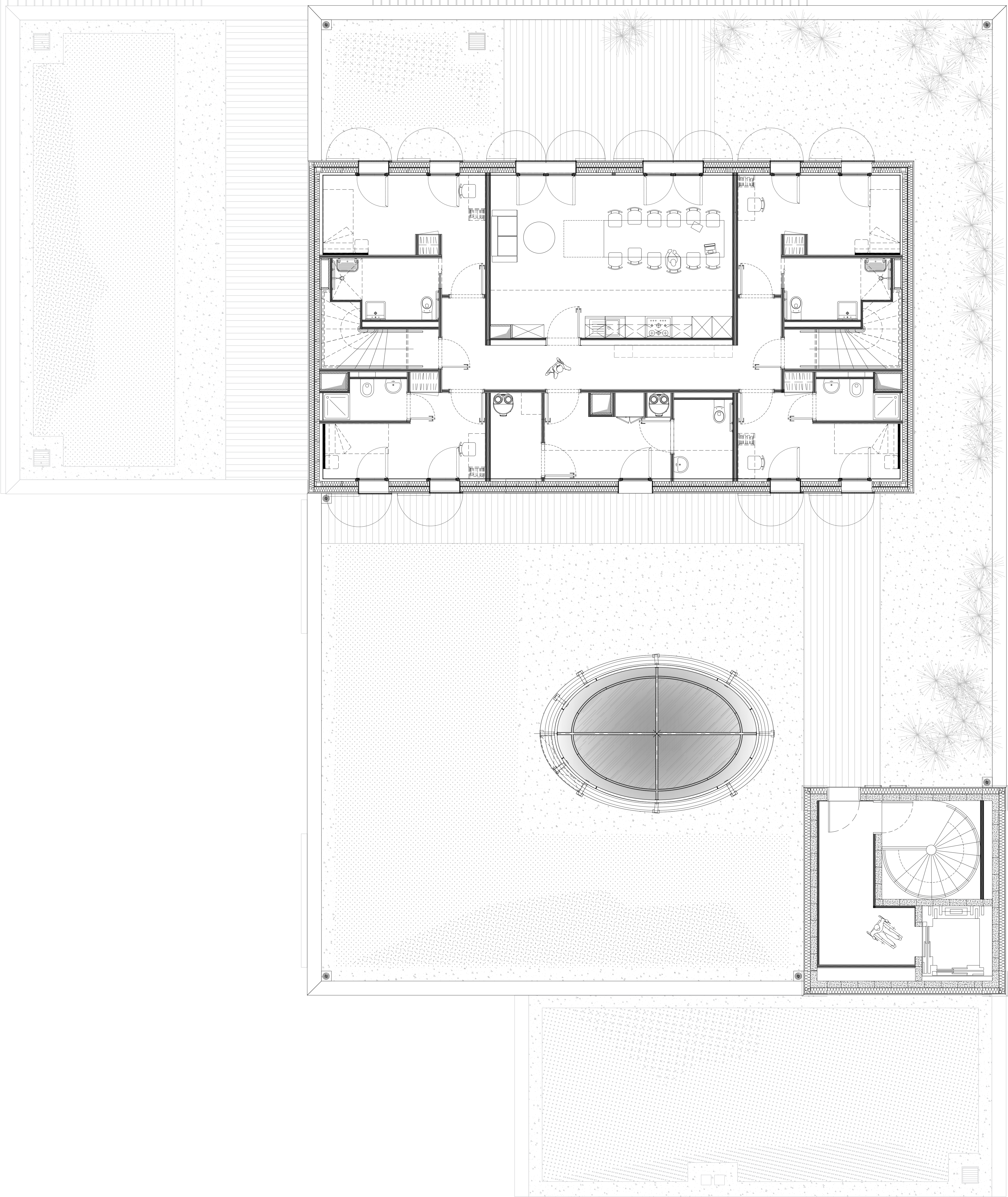
Plan du 3ème étage
