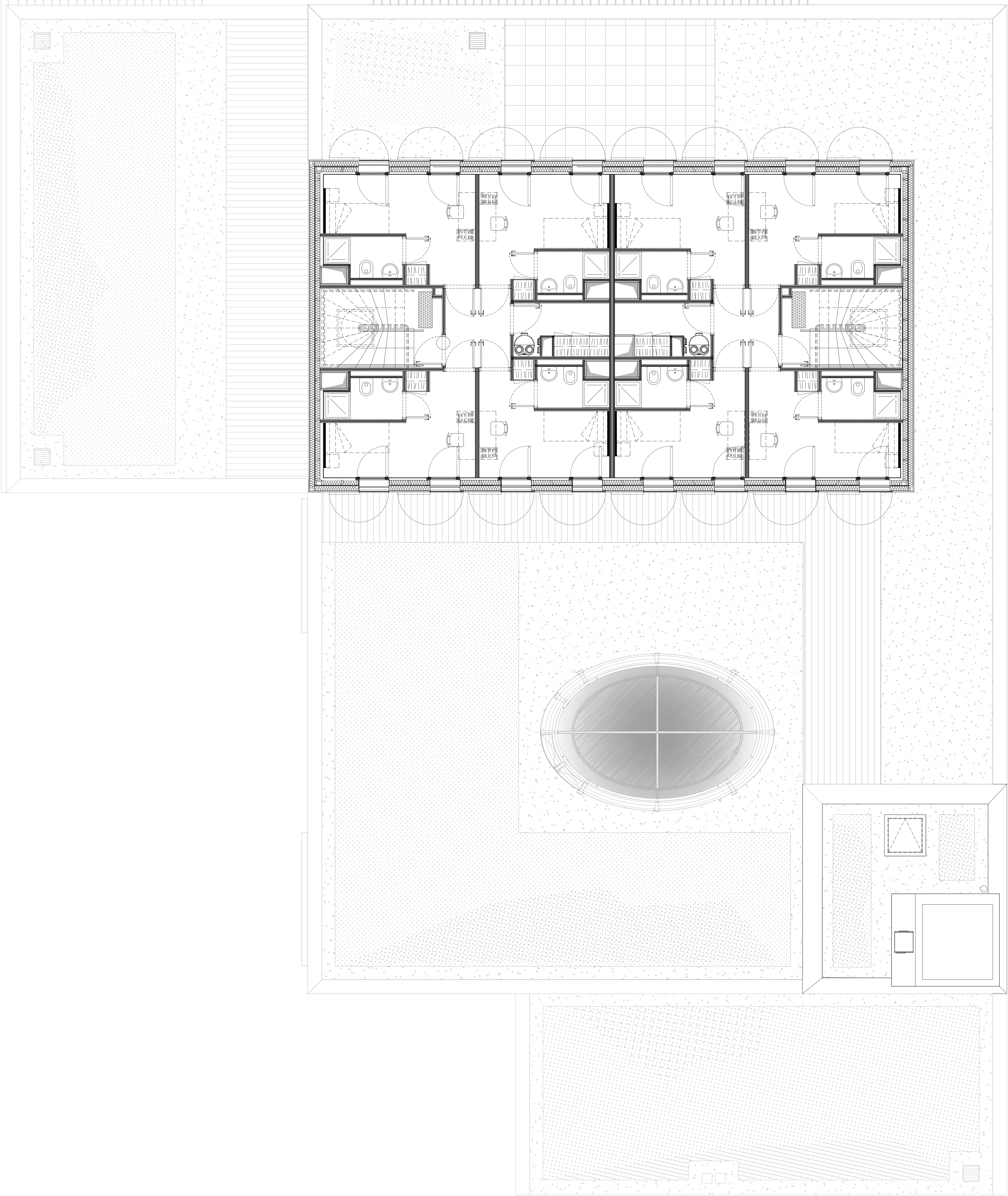
Plan du 4ème étage
