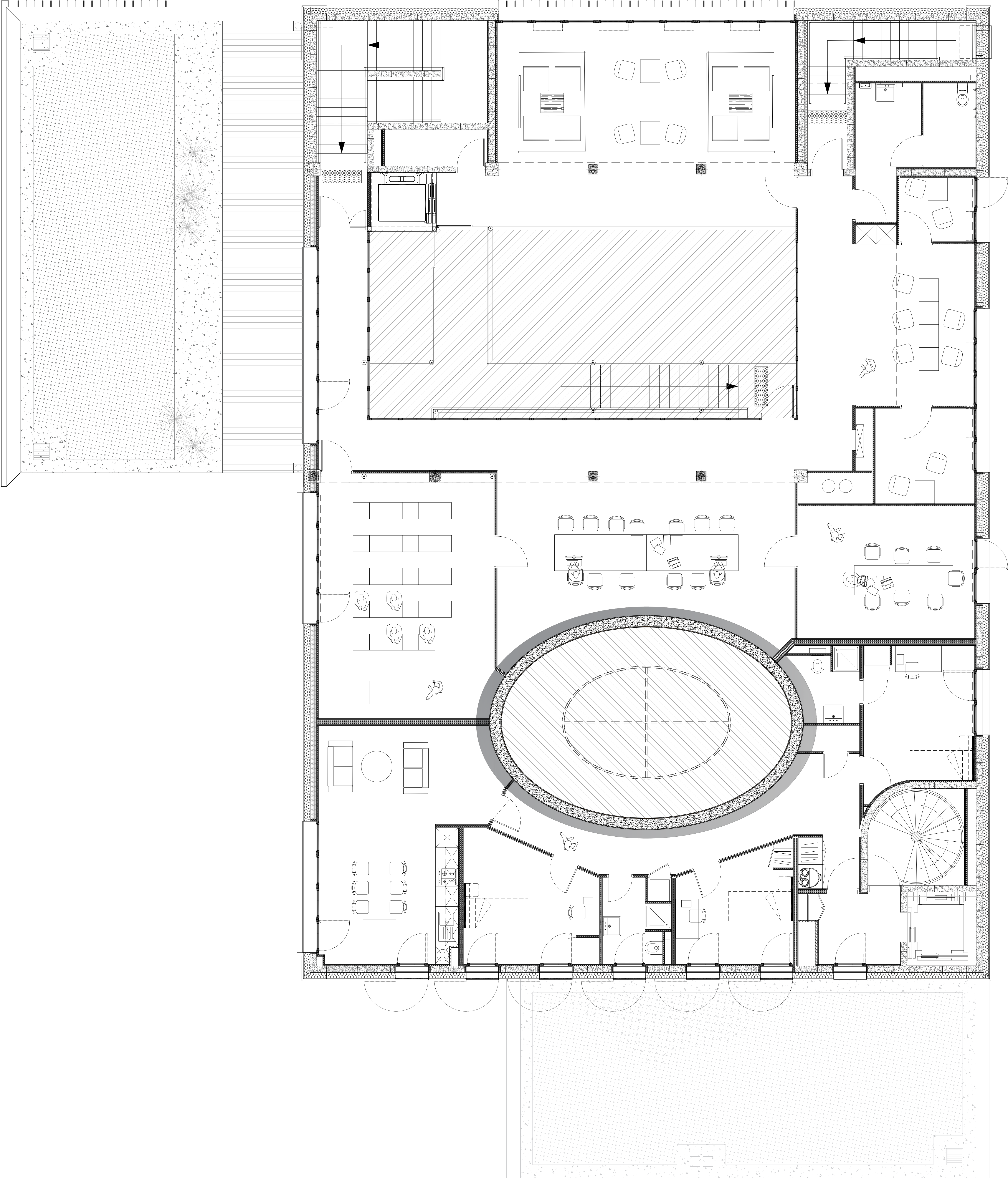
Plan du 2ème étage
