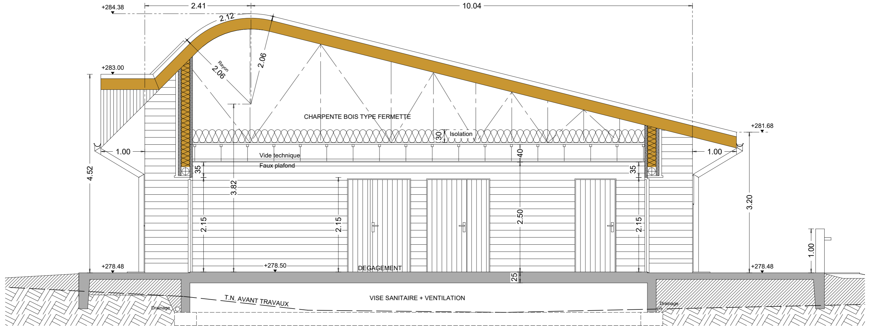
COUPE AA / DEGAGEMENT ECHELLE: 1/50
