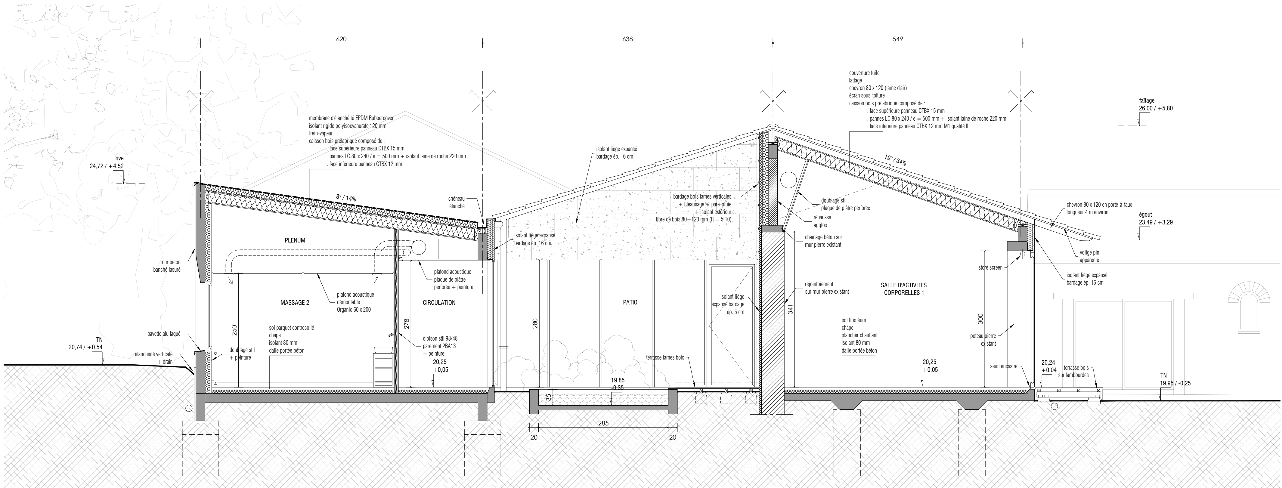
Coupe F-F
