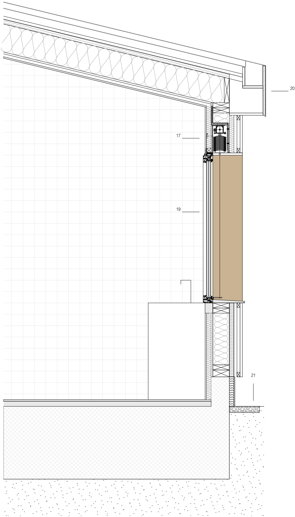
COUPE DETAIL MUR
