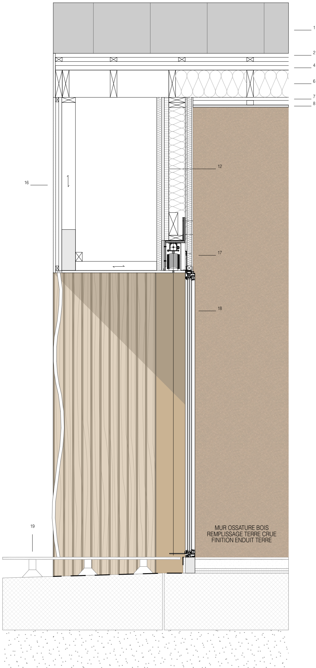
COUPE DETAIL TOITURE
