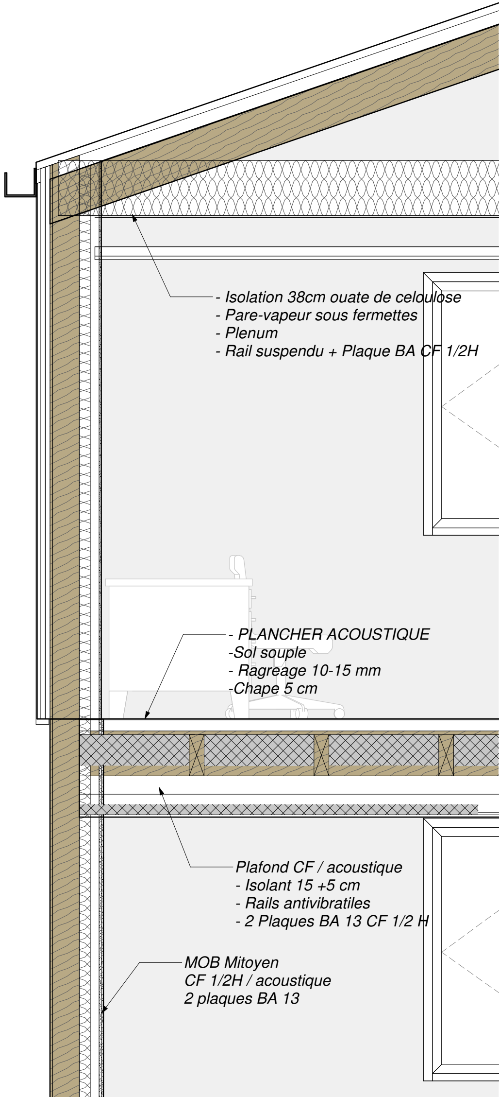
COUPE DETAIL COMPOSITION PAROIS - T3 SUPERPOSES
