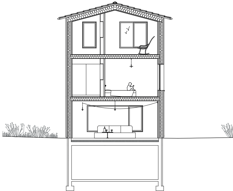
Coupe transversale AA 1:100°
