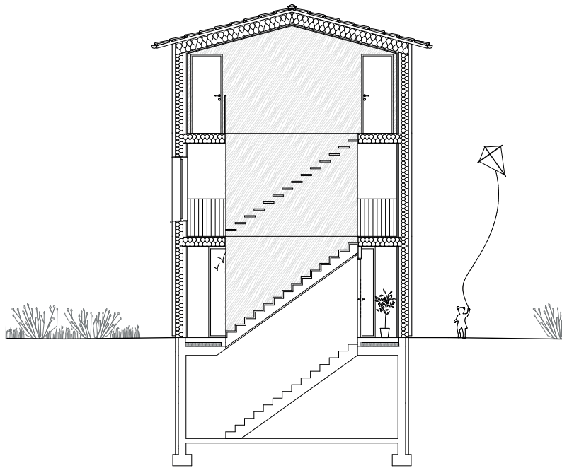
Coupe transversale BB 1:100°
