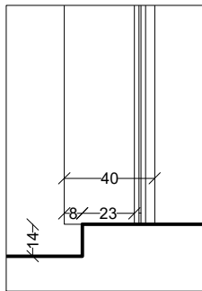
COUPE AA' Echelle 1.30
