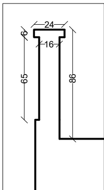
COUPE BB' Echelle 1.30
