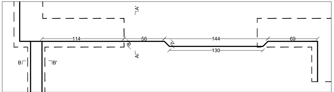
DETAIL Plan de la dalle au niveau du sol Echelle 1.30
