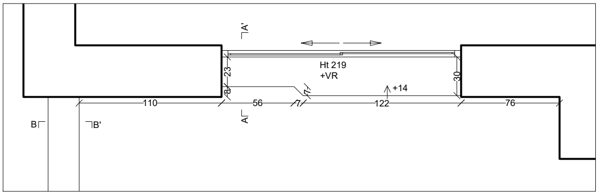
DETAIL Plan à + 100 Echelle 1.30
