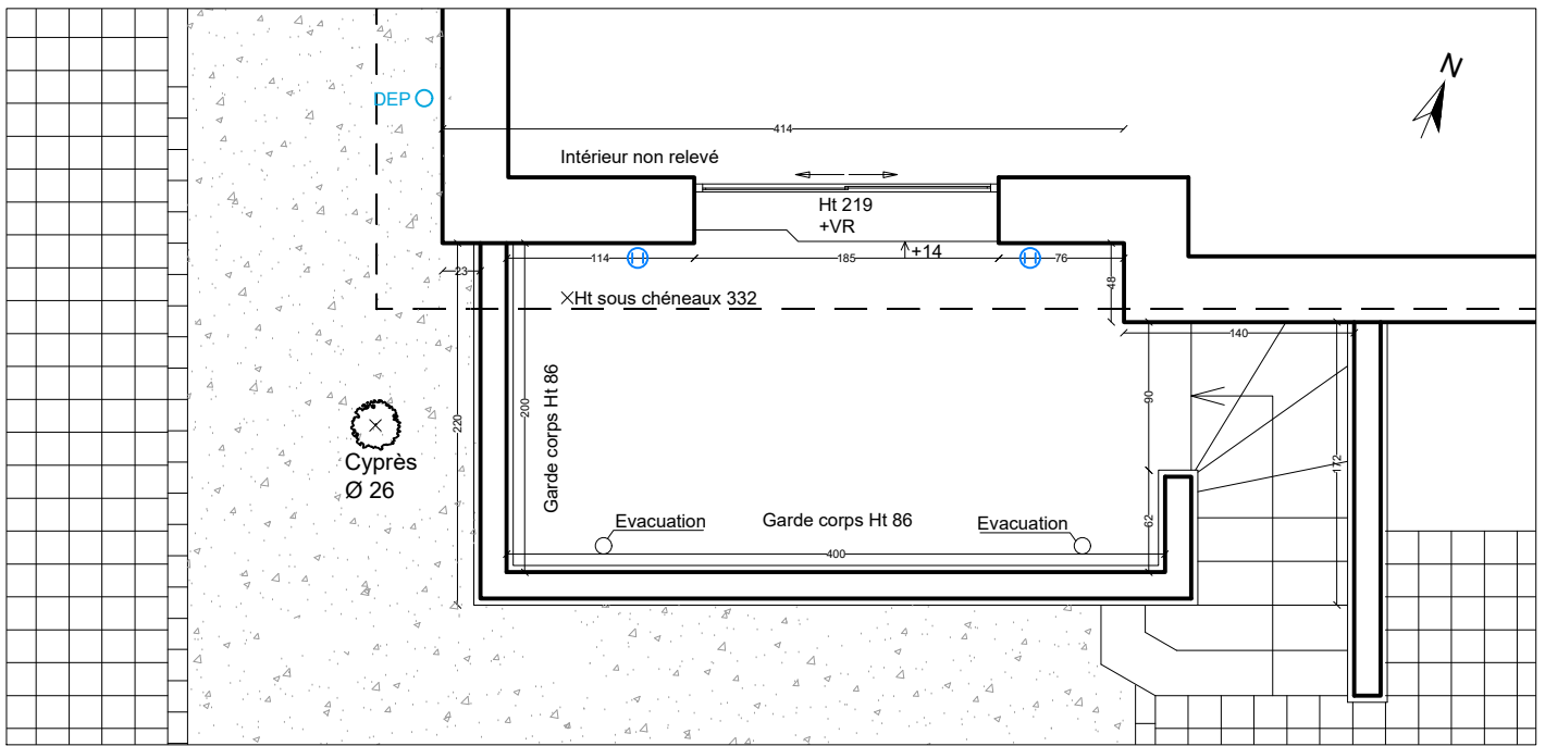
PLAN R+1 Echelle 1.50
