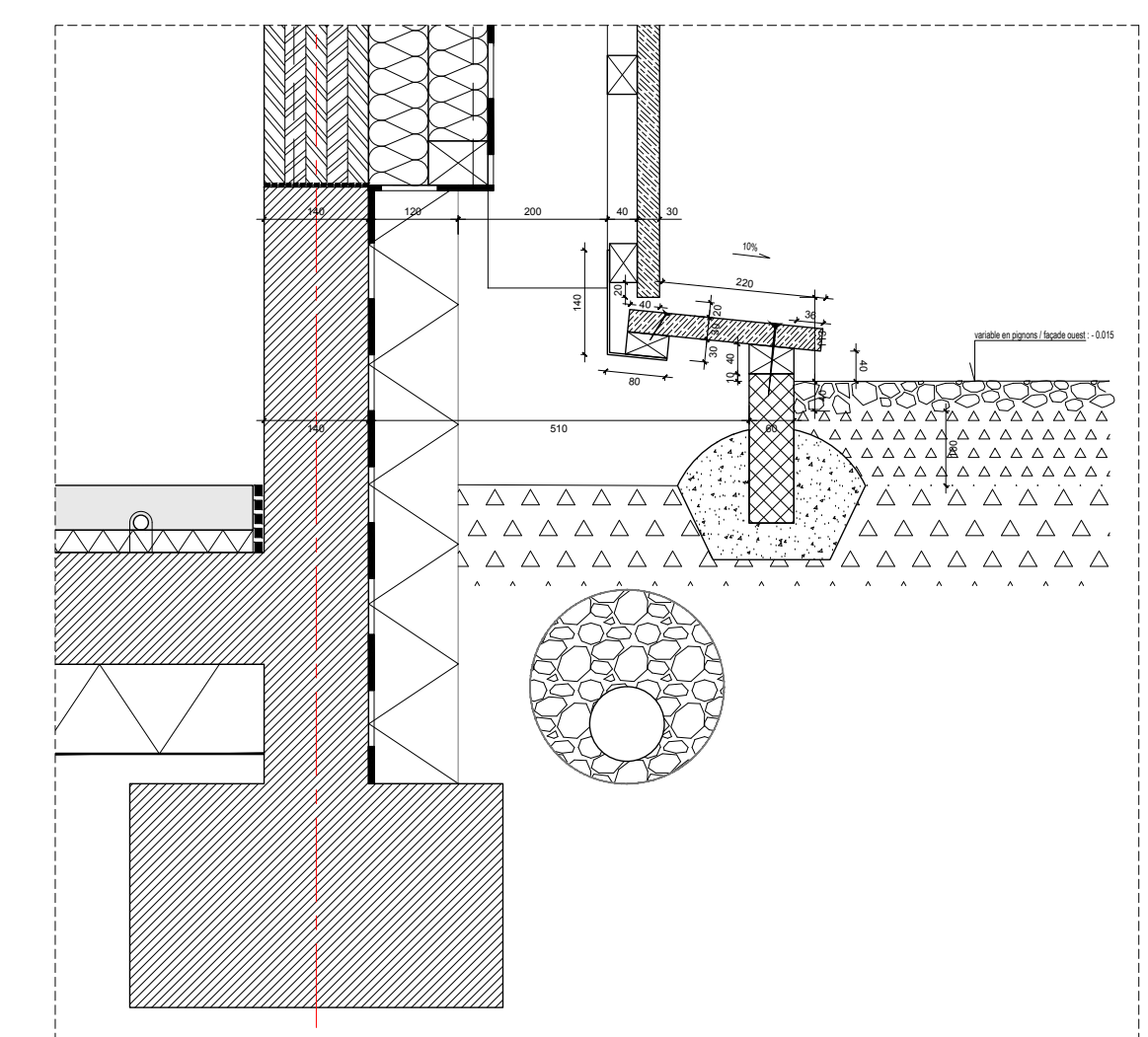
DETAIL PIED DE FACADE PIGNON SUD 1/10e
