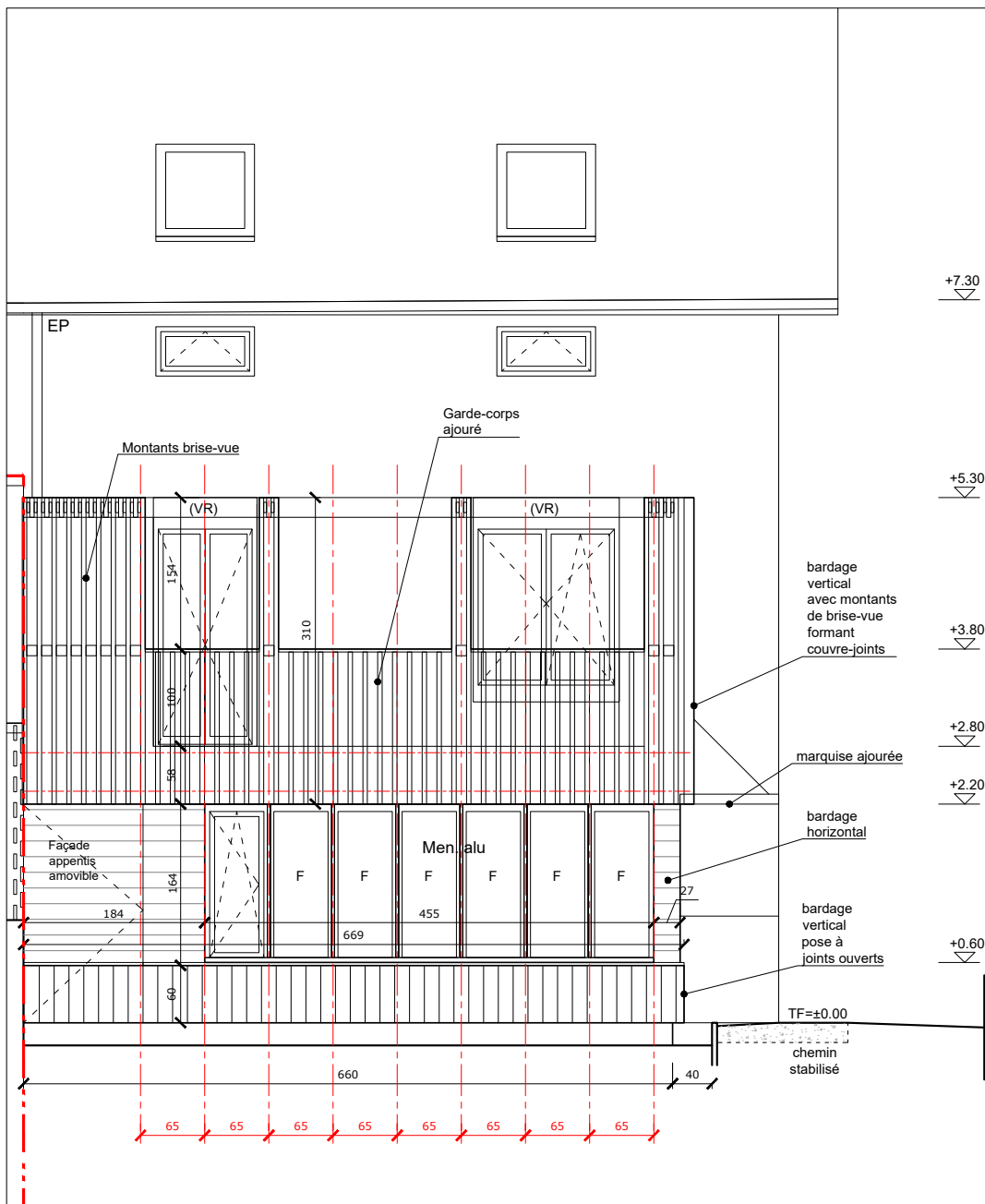
FACADE EST
