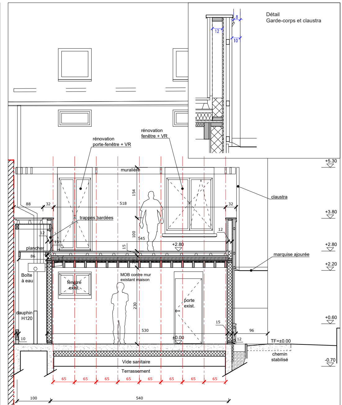
COUPE LONGITUDINALE appentis + atelier
