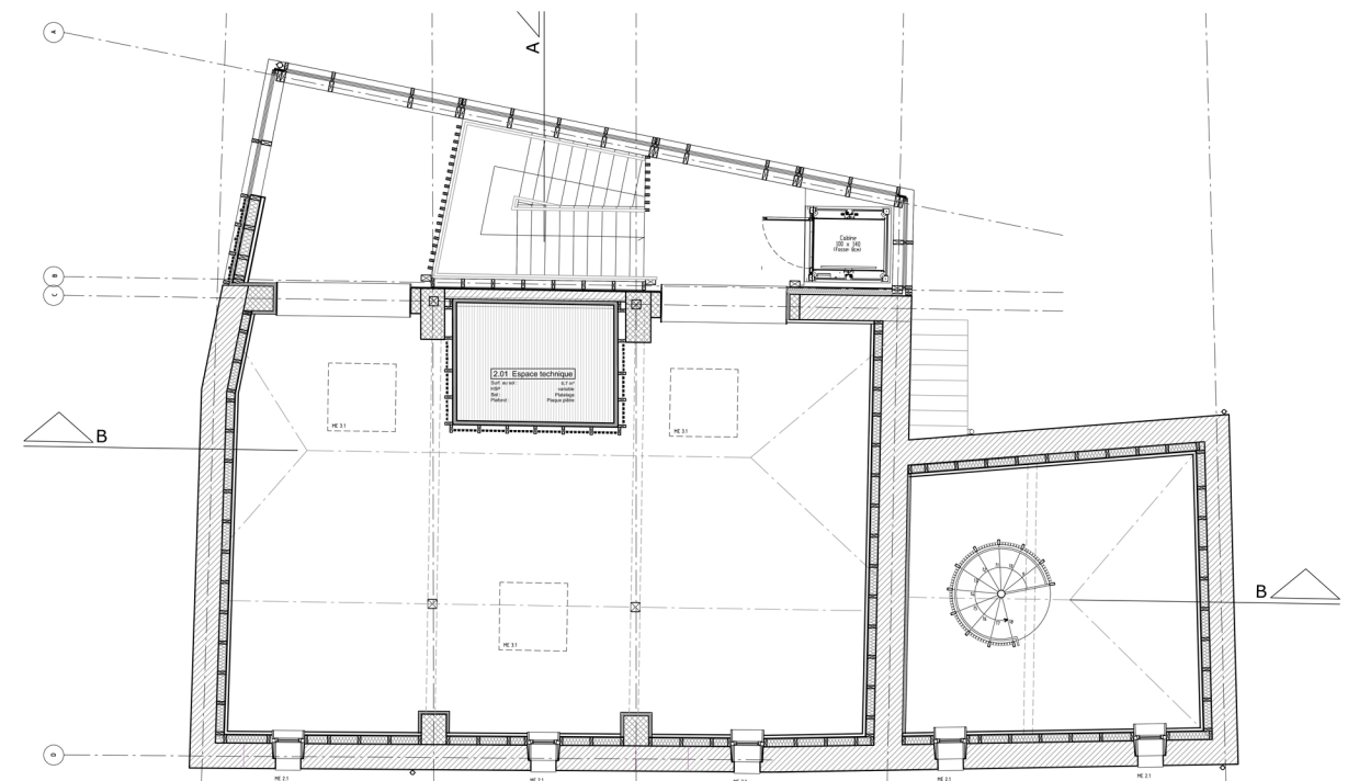
PLAN R+2 CTA Echelle 1/50
