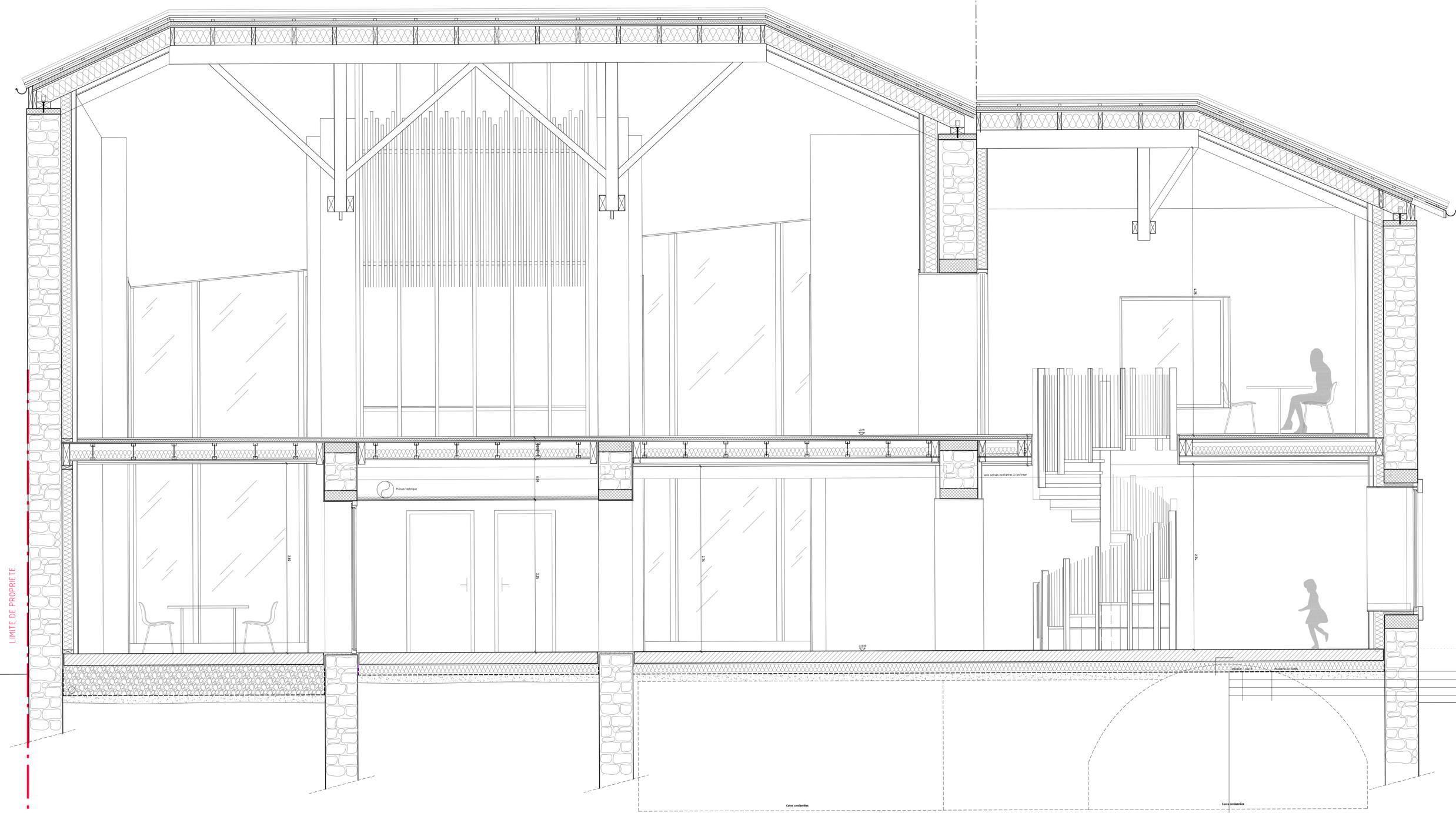
COUPE LONGITUDINALE Echelle 1/20
