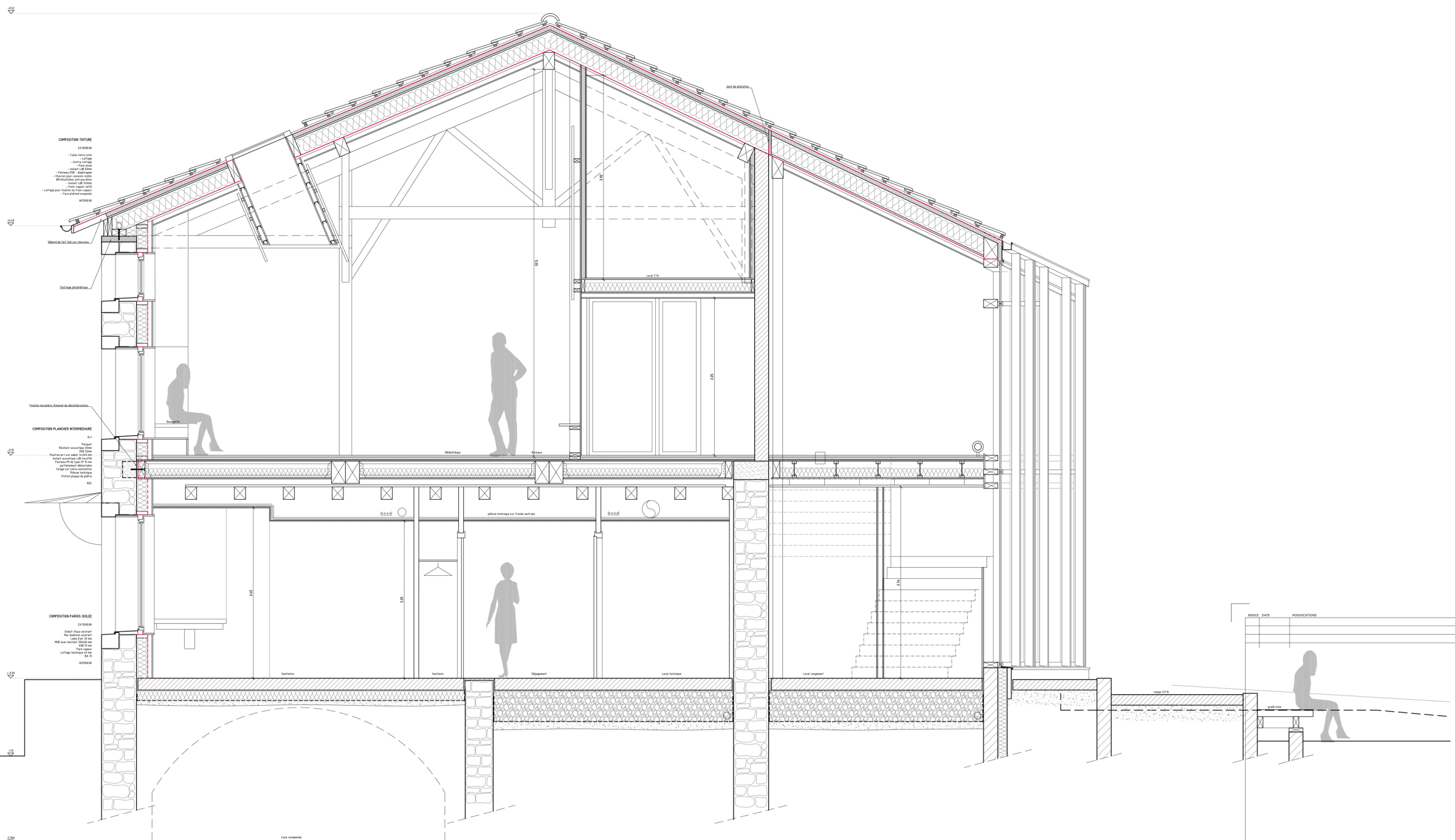
COUPE TRANSVERSALE Echelle 1/20
