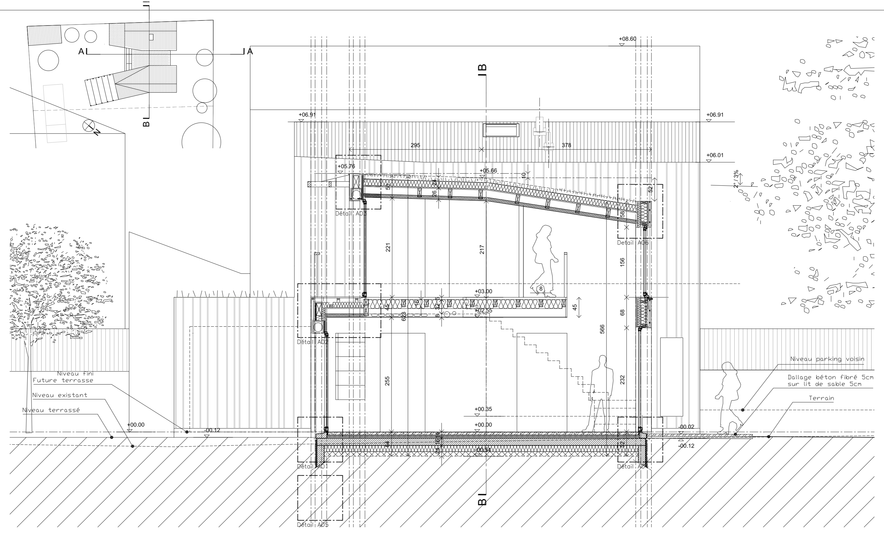
Coupe AA Coupe longitudinale - Projet
