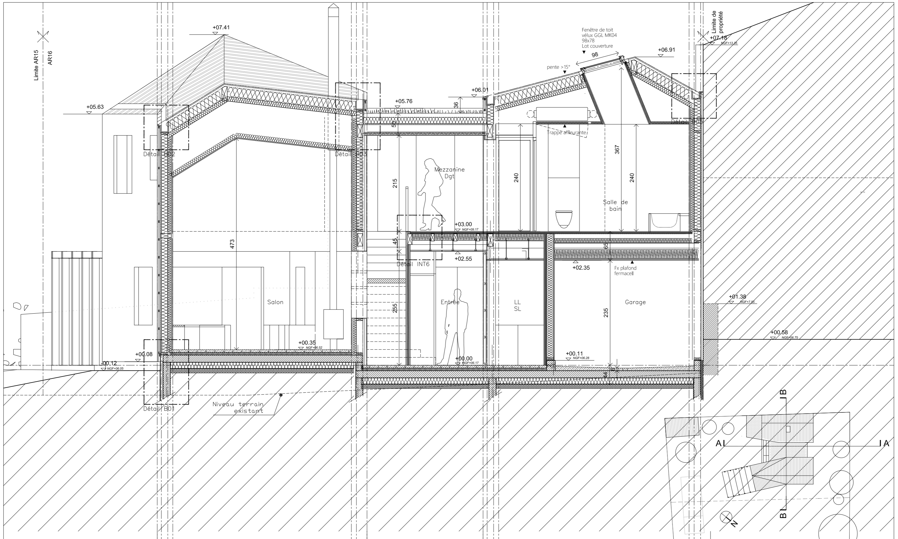
COUPE BB Coupe transversale - Projet
