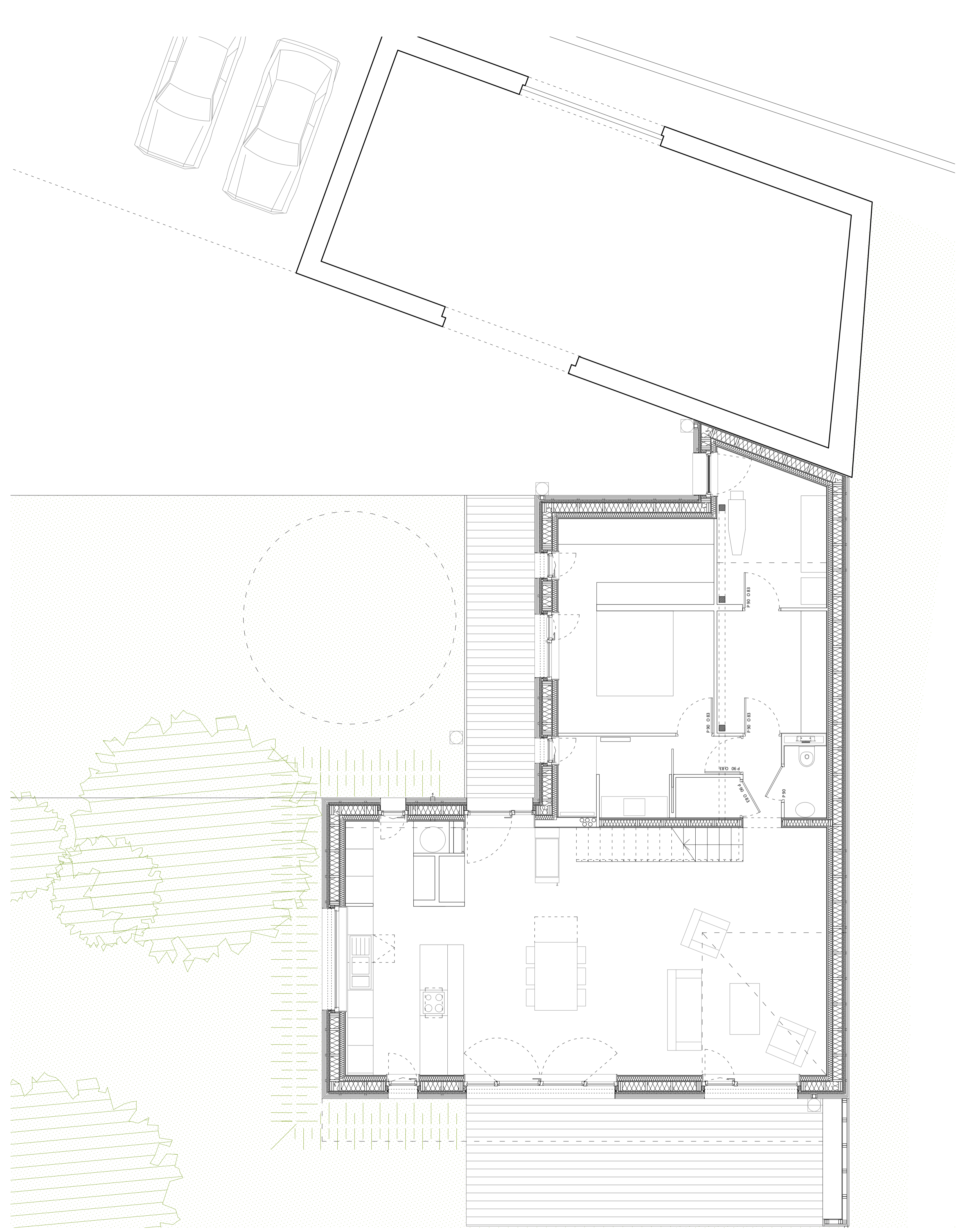
PLAN DU REZ-DE-CHAUSSEE
