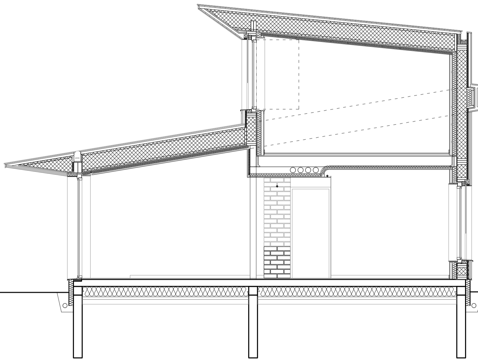
COUPE NORD -SUD : CHAMBRES - SEJOUR
