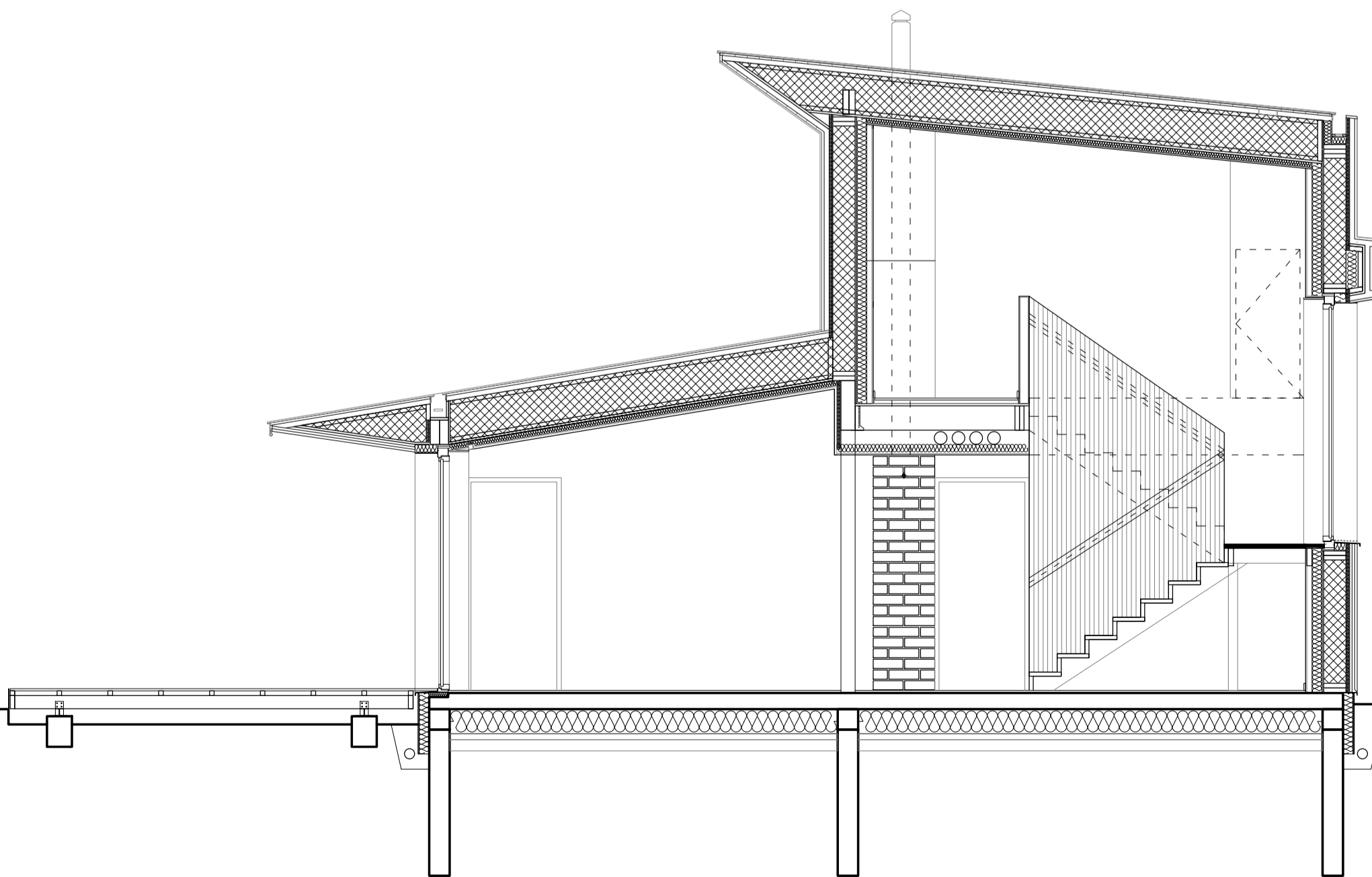
COUPE NORD -SUD : SALLE A MANGER ESCALIER
