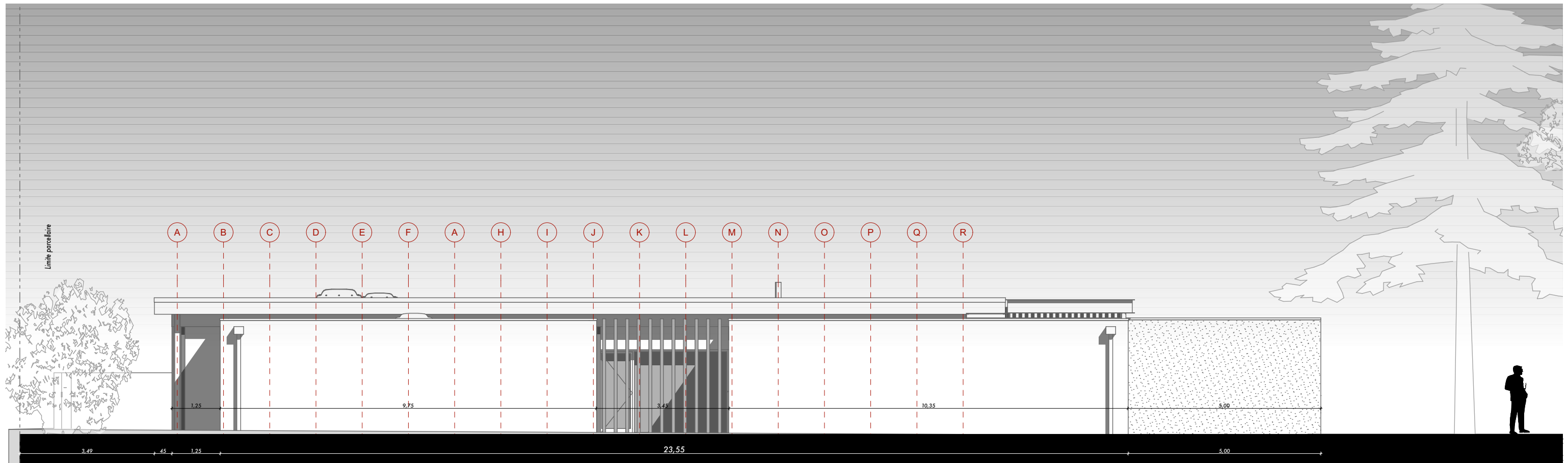
ÉLEVATION FAÇADE OUEST 1/100
