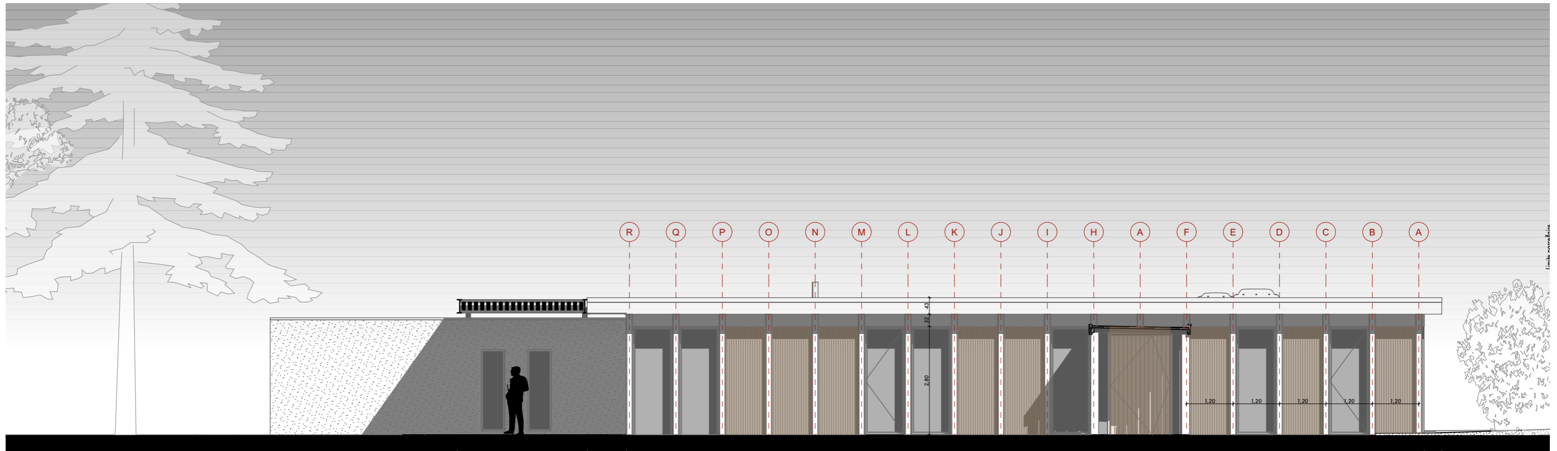
ÉLEVATION FAÇADE EST 1/100
