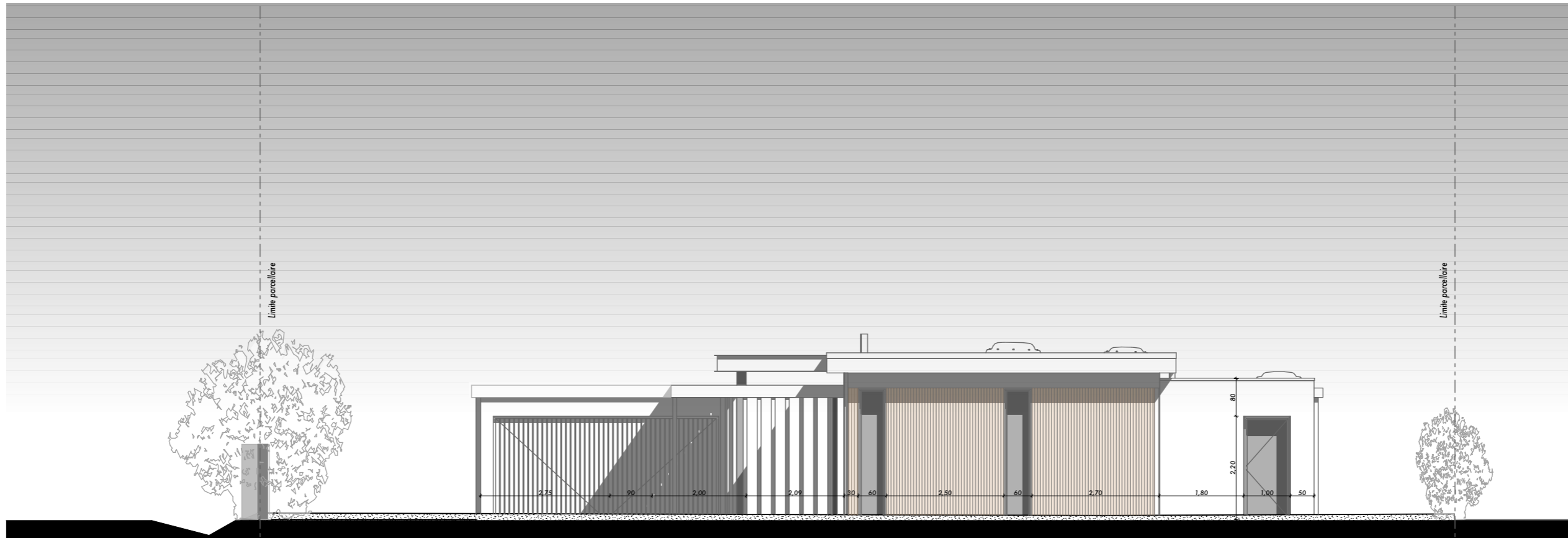
ÉLEVATION FAÇADE NORD 1/100
