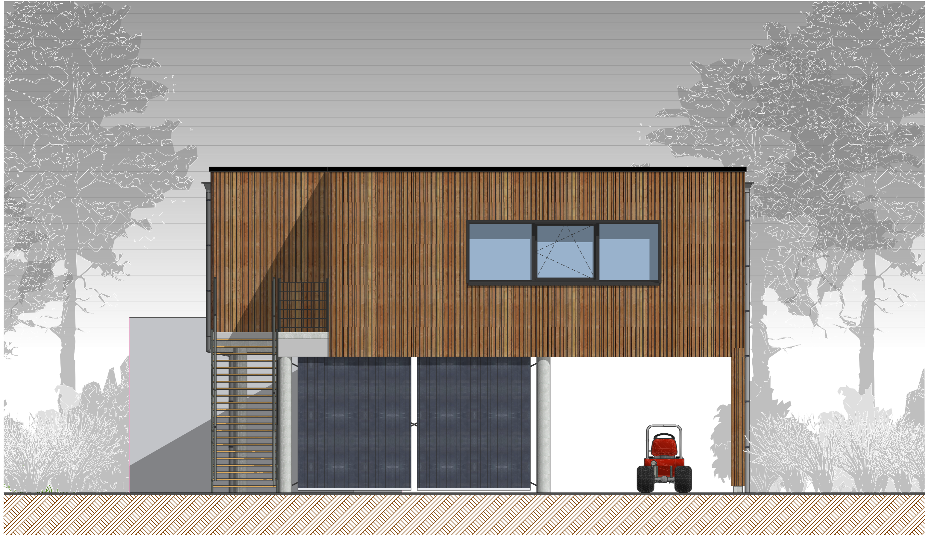
ÉLEVATION FAÇADE OUEST 1/50
