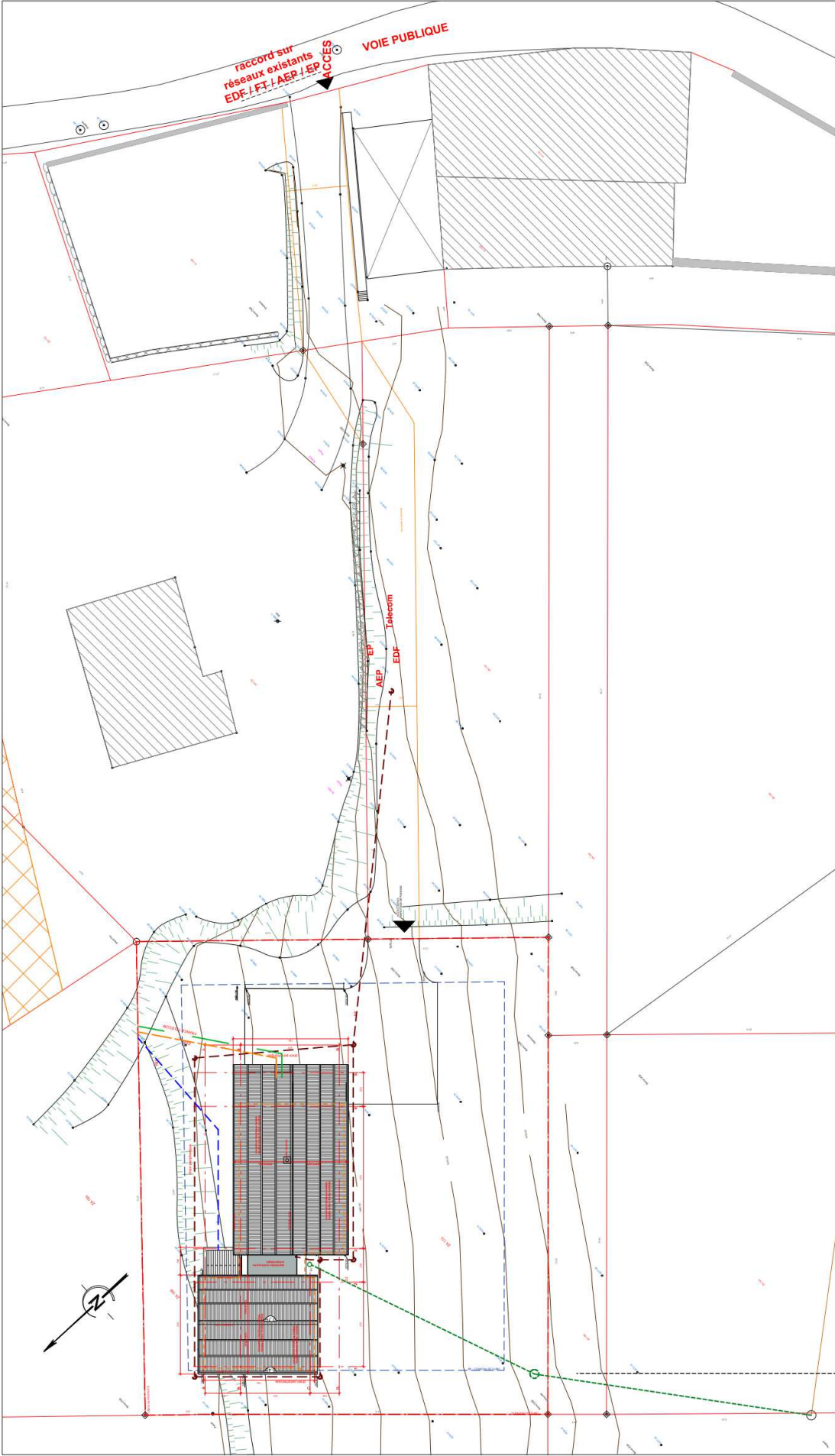
01.2 - PLAN DE MASSE RESEAUX - 1/250
