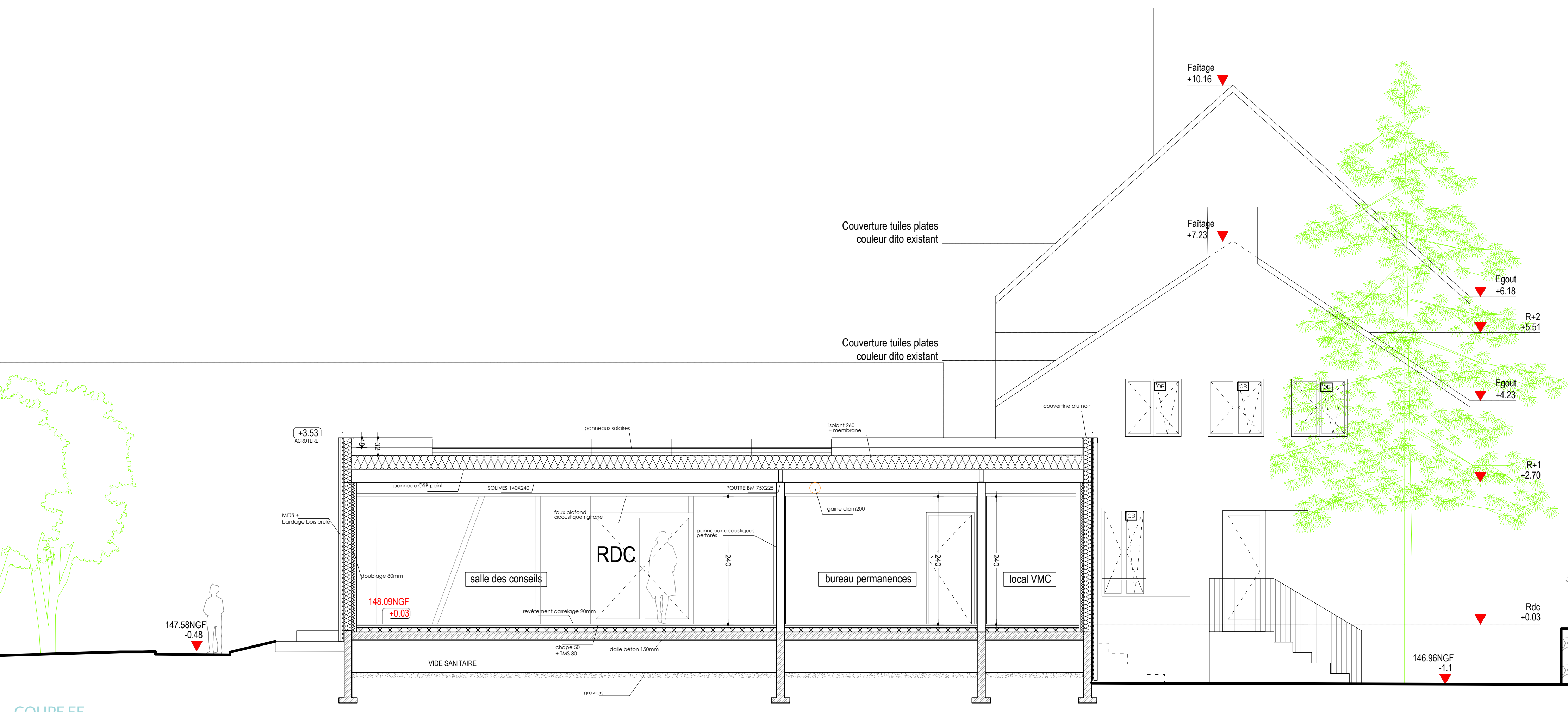
COUPE EE
