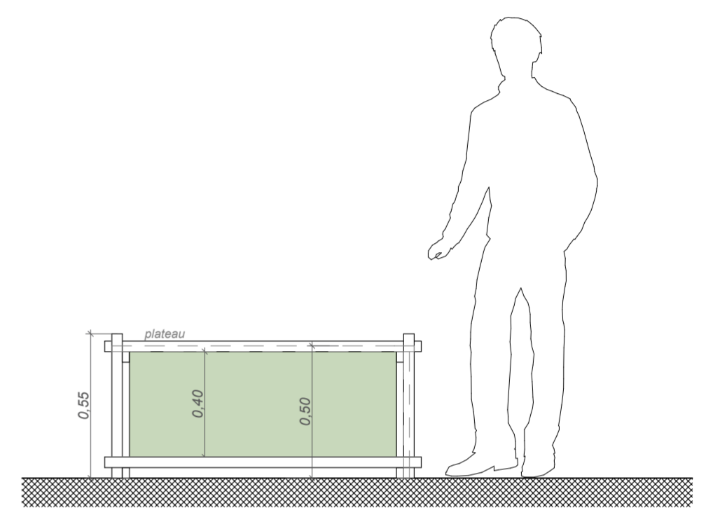
Elévation - module 1 et 6
