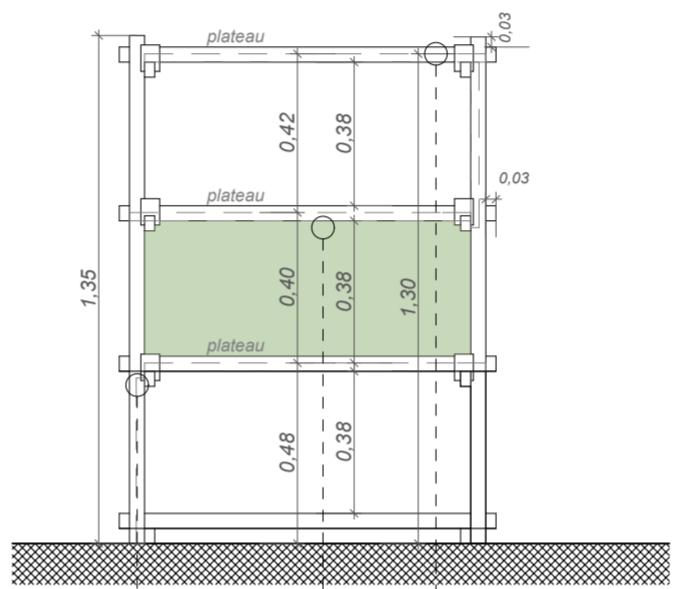
Elévation - module 2
