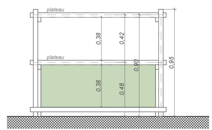
Elévation - module 4
