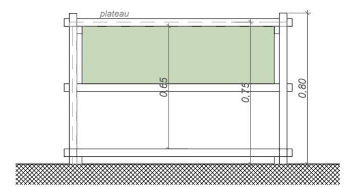
Elévation - module 3 et 5
