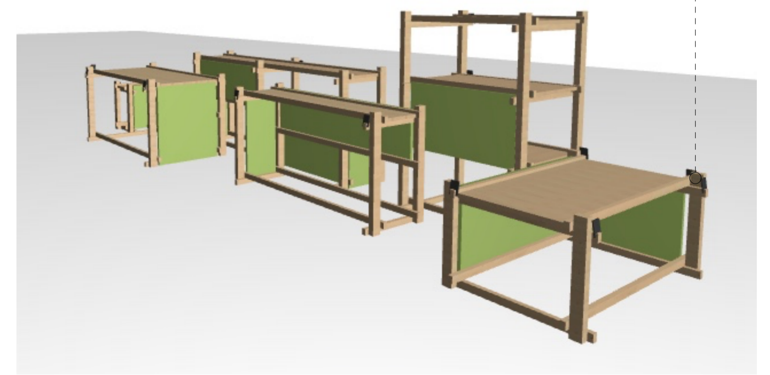
Vue 3D
