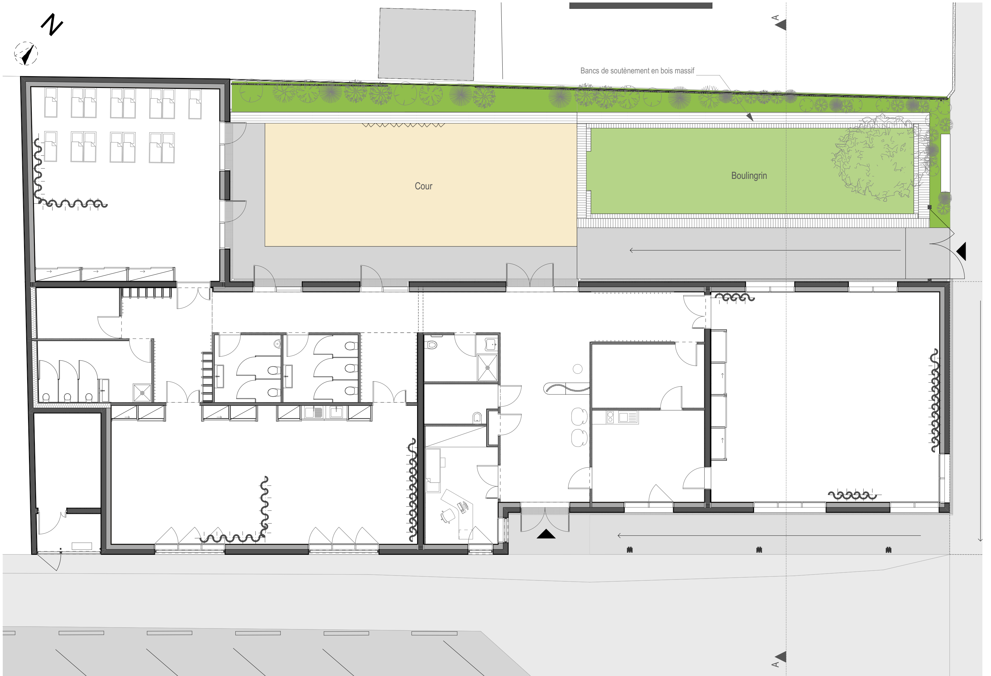
Plan RDC
