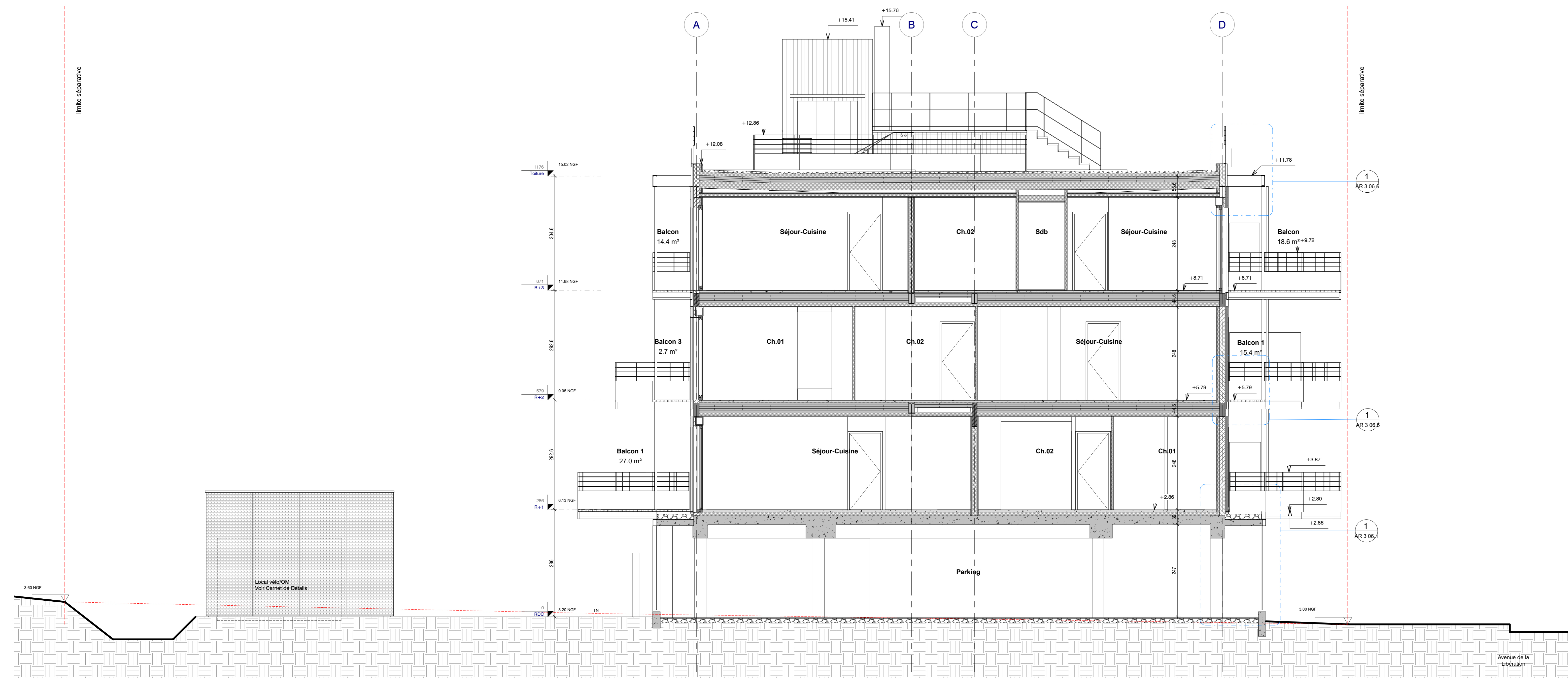
2- Coupe BB'
