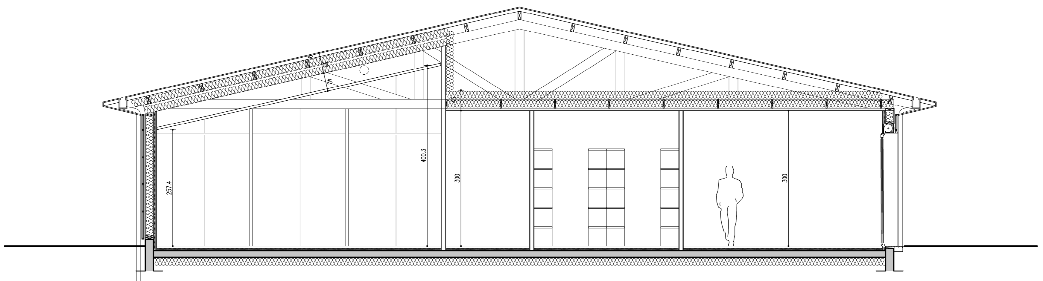
COUPE D
