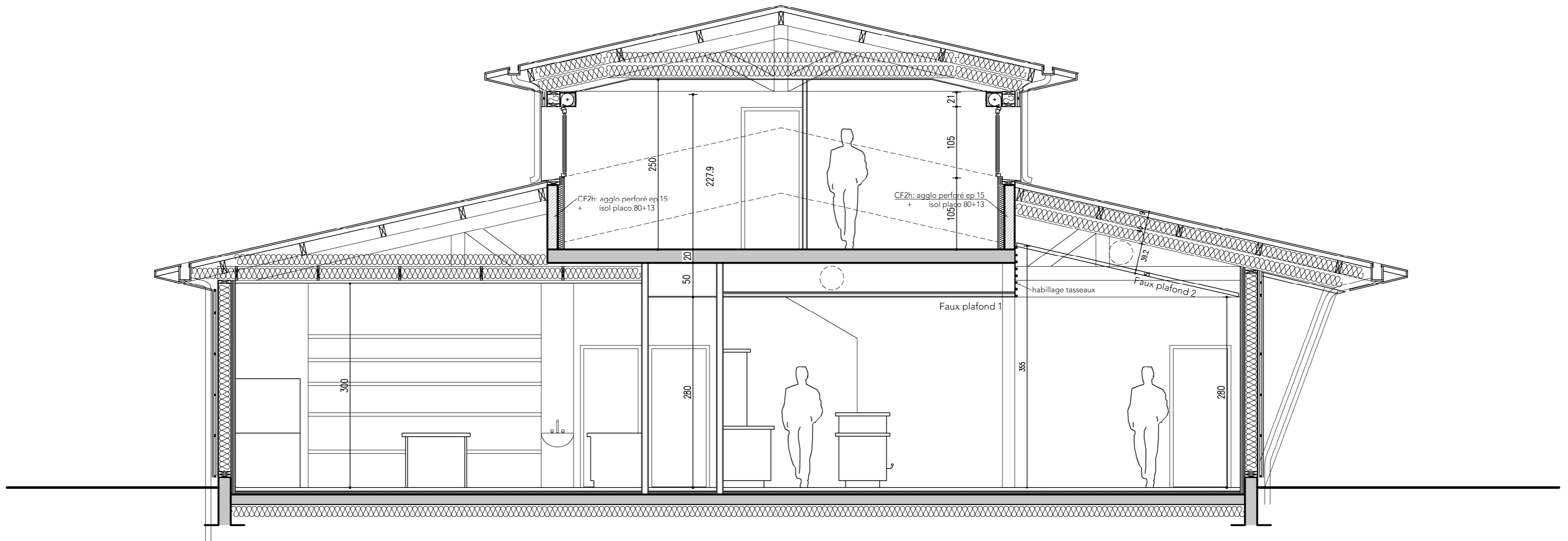
COUPE B
