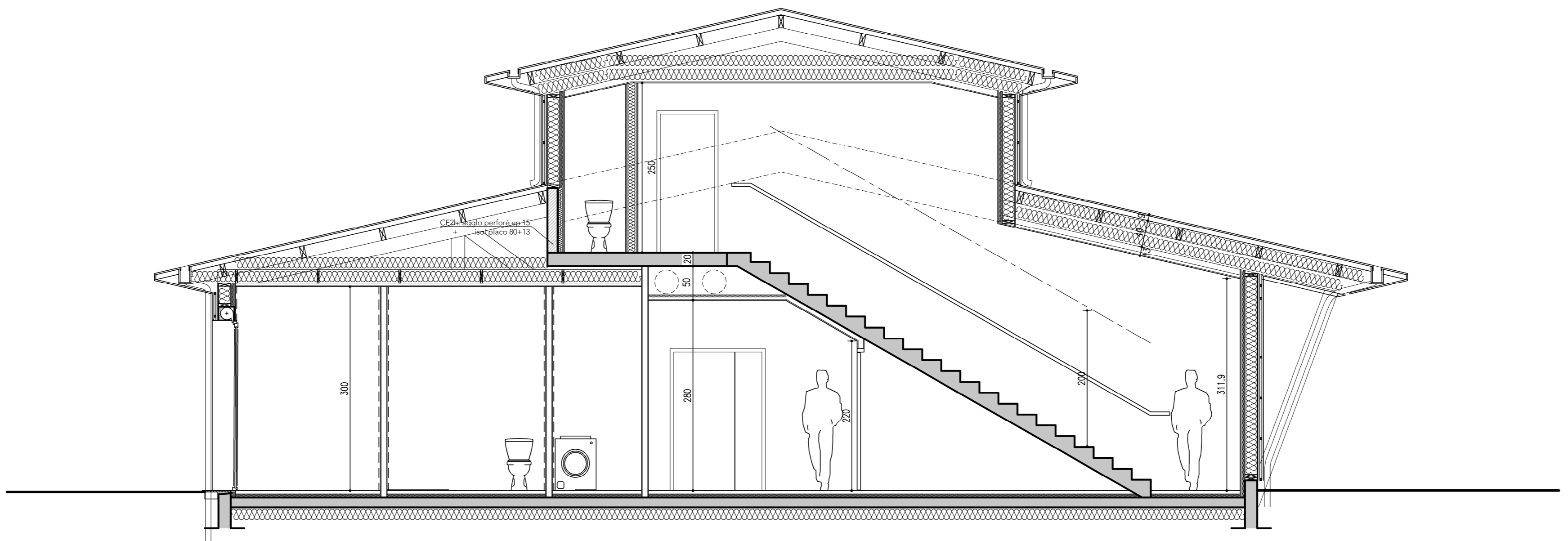
COUPE C
