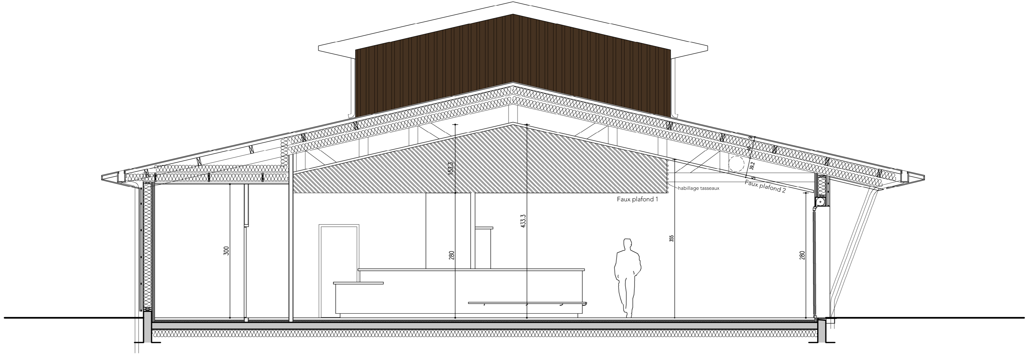
COUPE A
