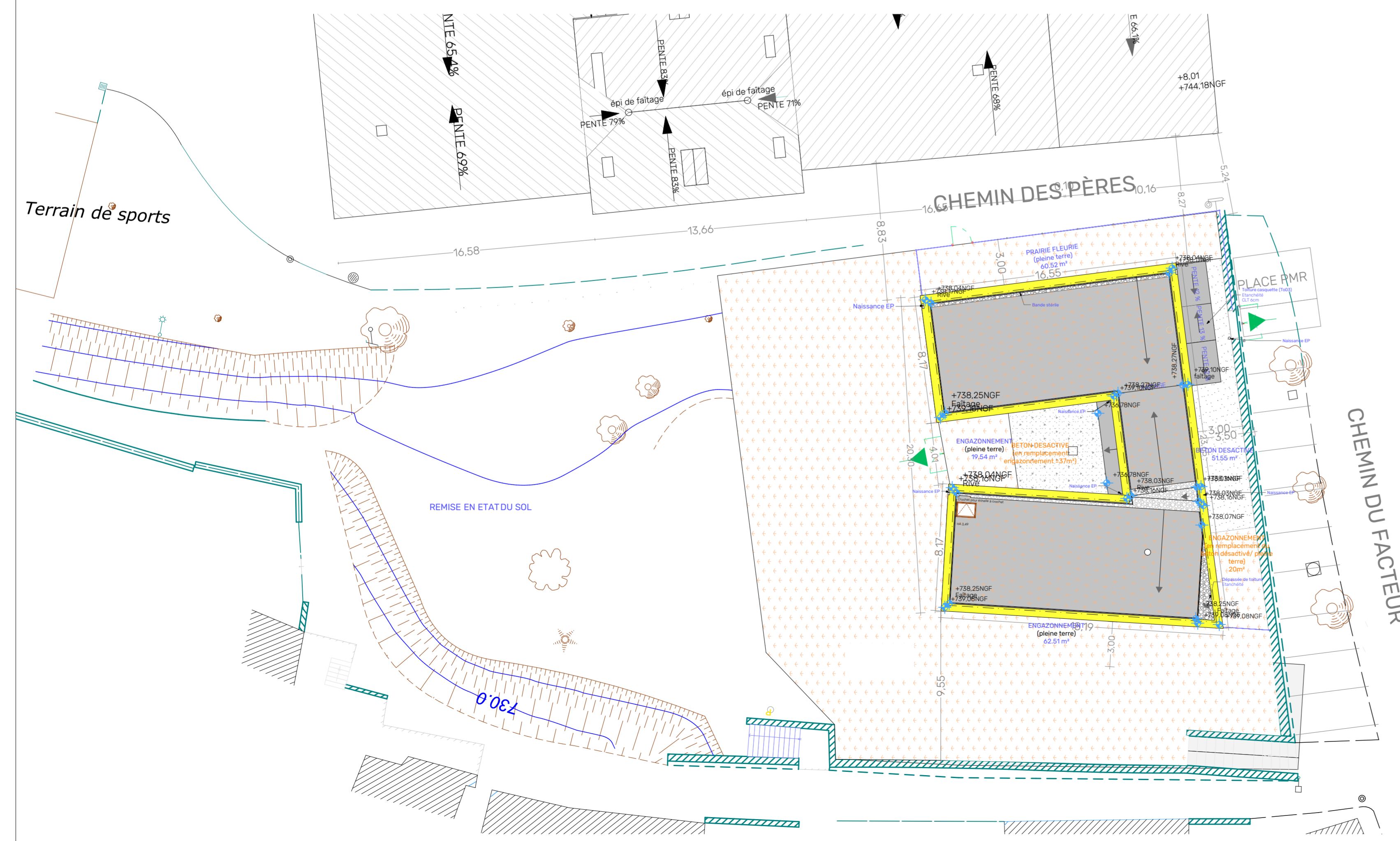
PLAN - MASSE échelle 1:200
