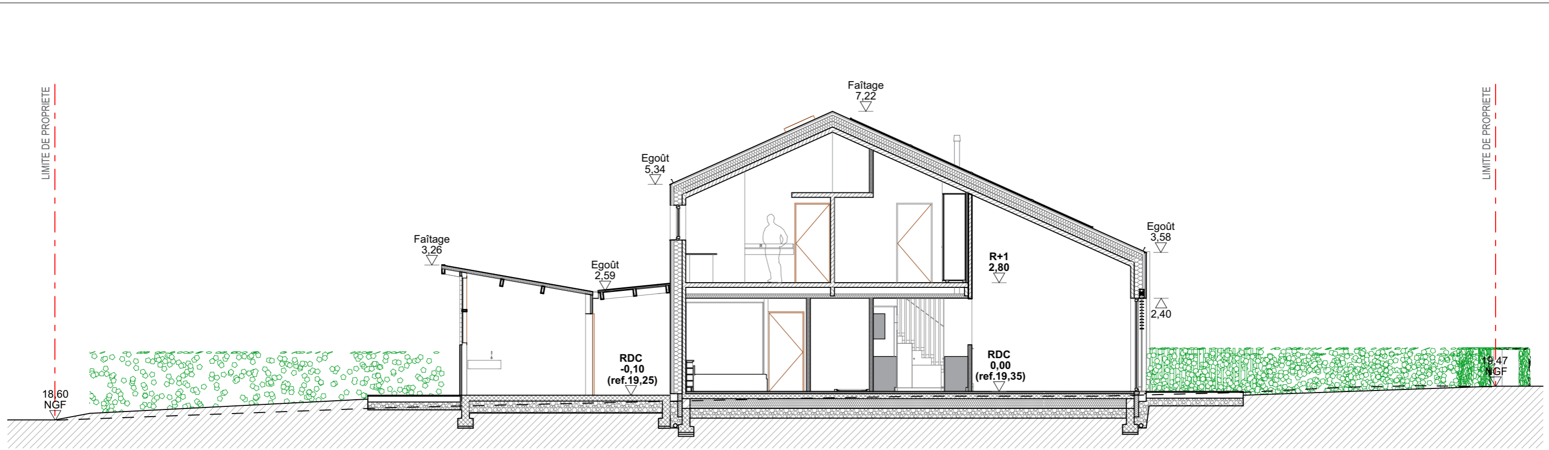
Coupe AA'
