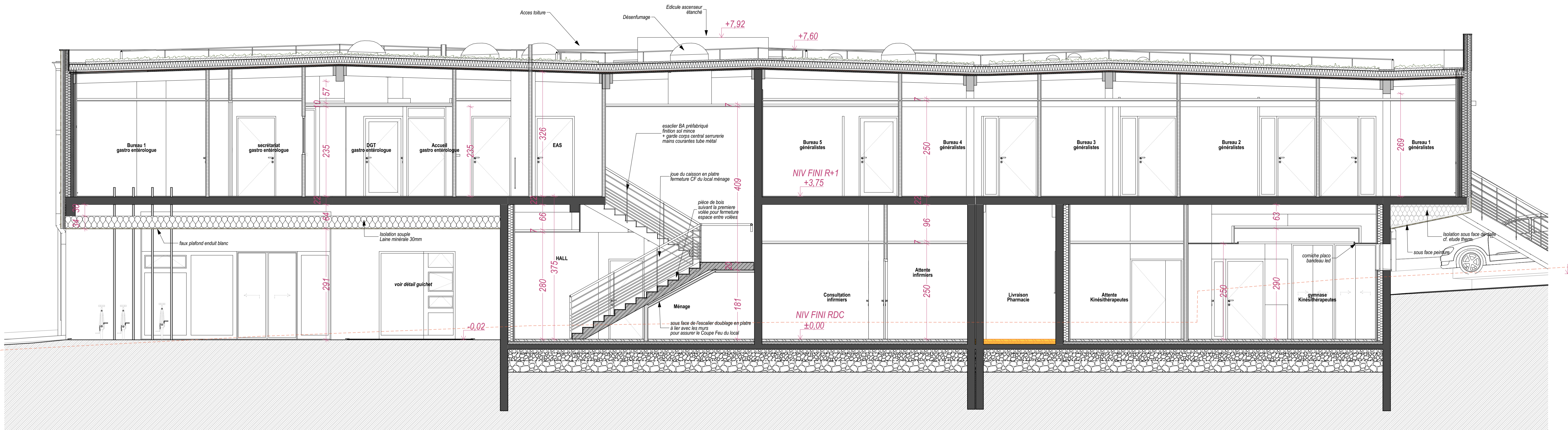
COUPE EE
