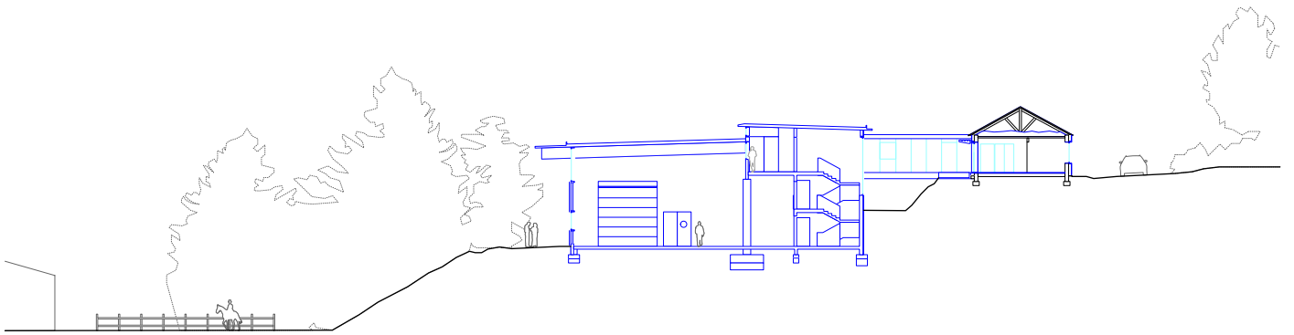
Coupe T - 1/500
