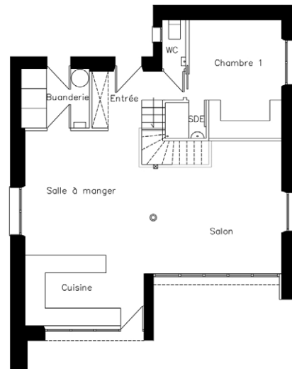
Plan rez-de-chaussée
