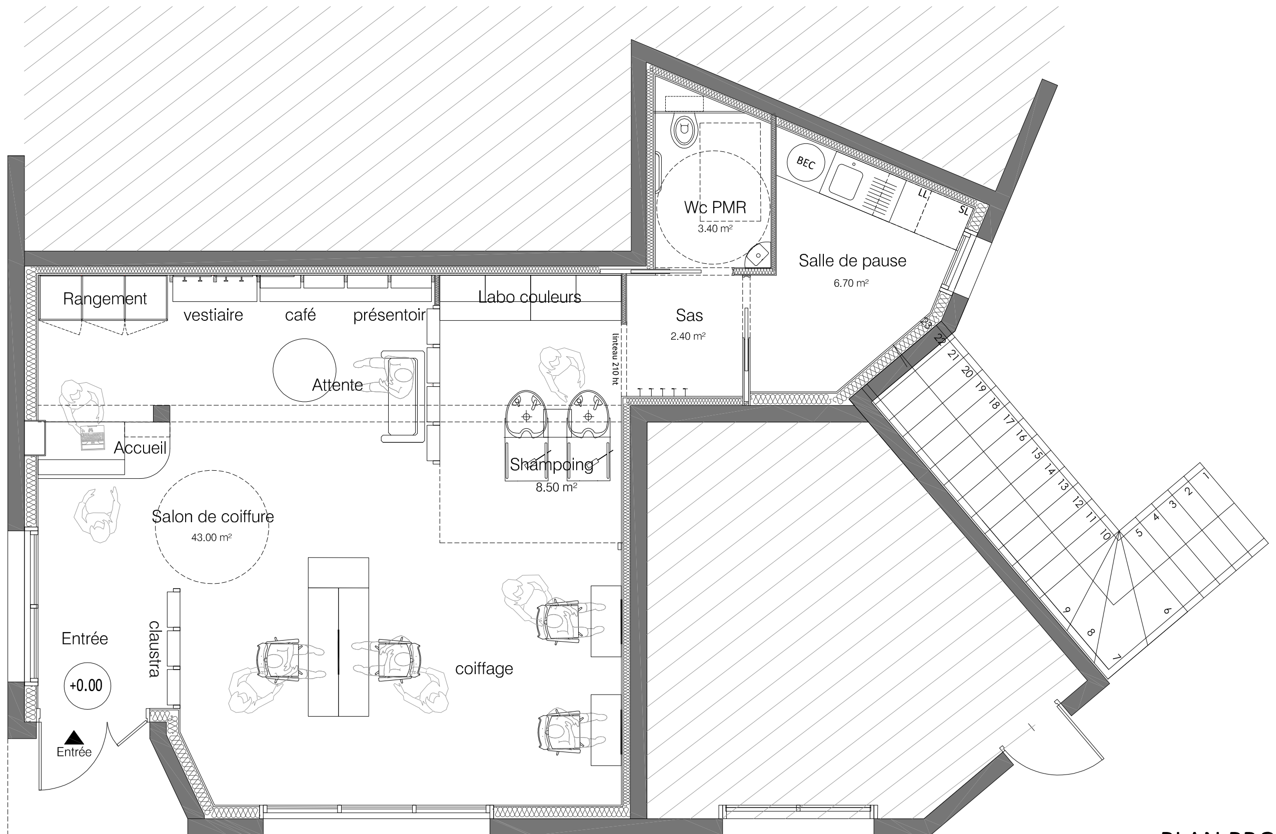
PLAN PROJET échelle : 1/50
