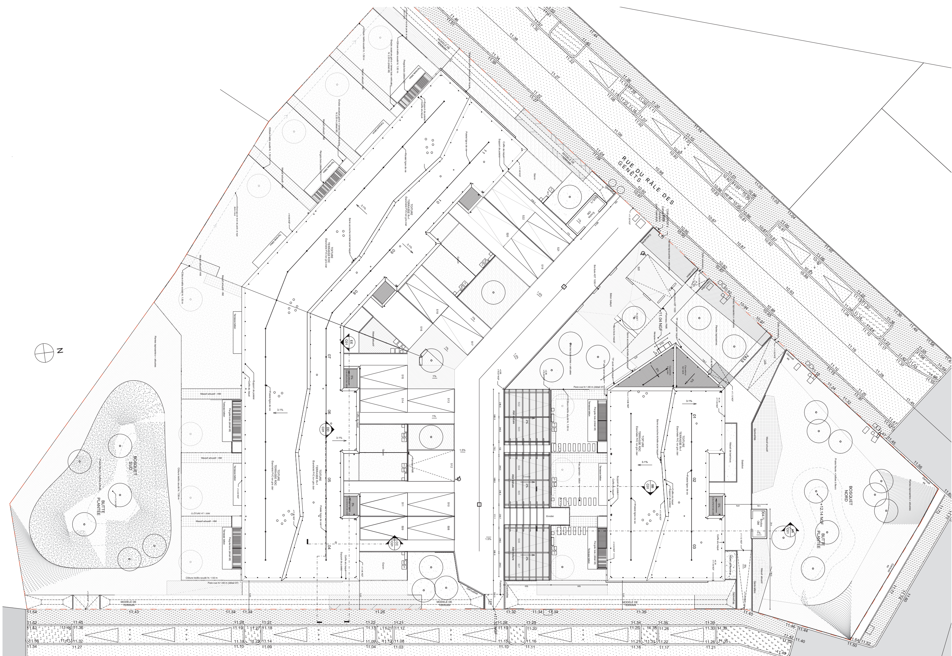
PLAN MASSE _ 1/250
