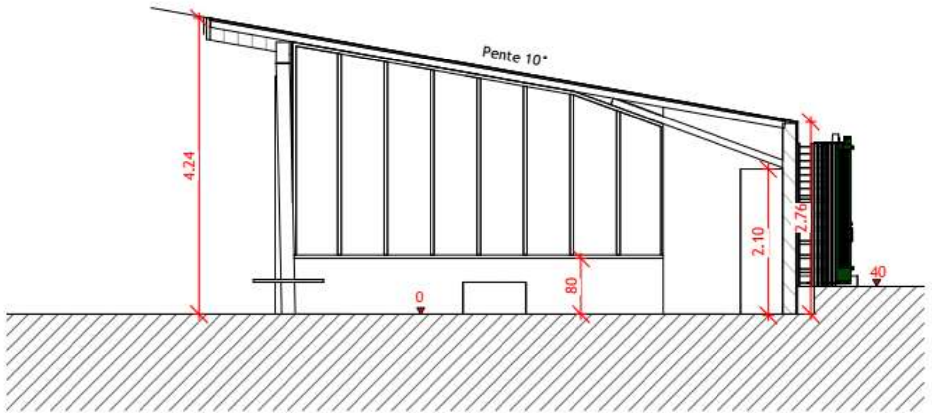
3 | Coupe A-A 1 : 75
