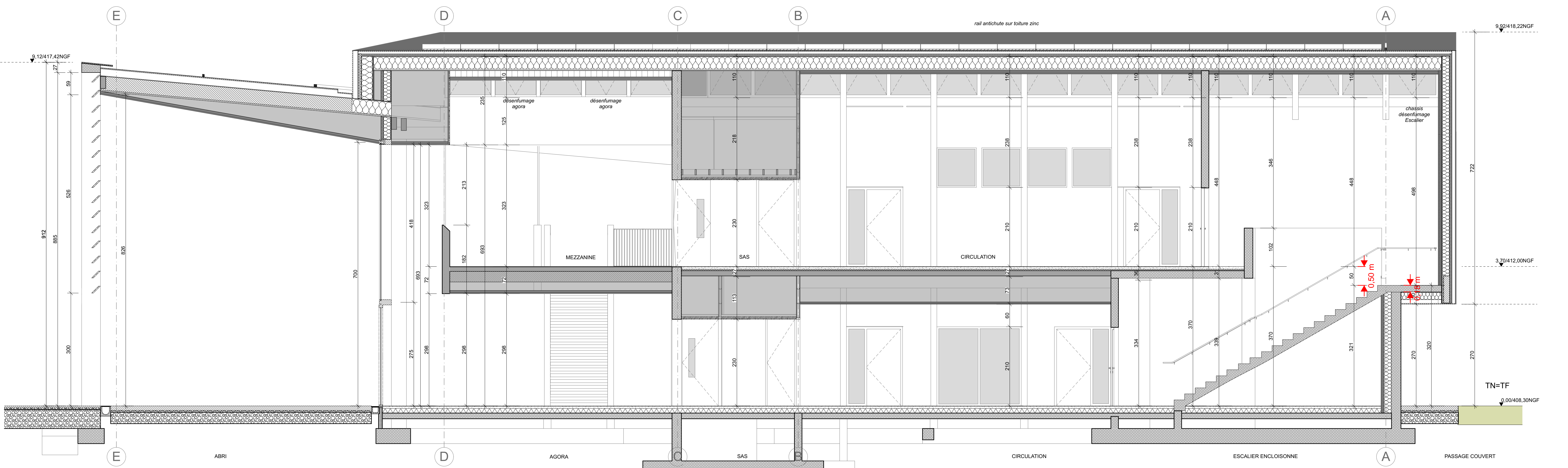
D - Coupe bloc 3 / préau Nord
