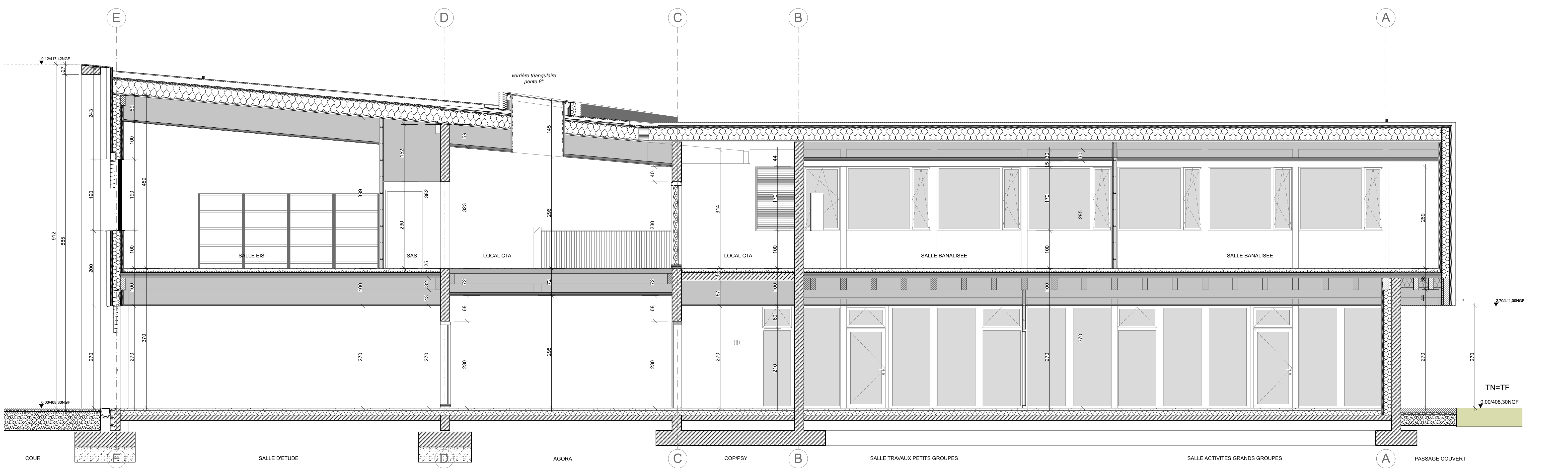
E - Coupe blocs 2/5 Nord
