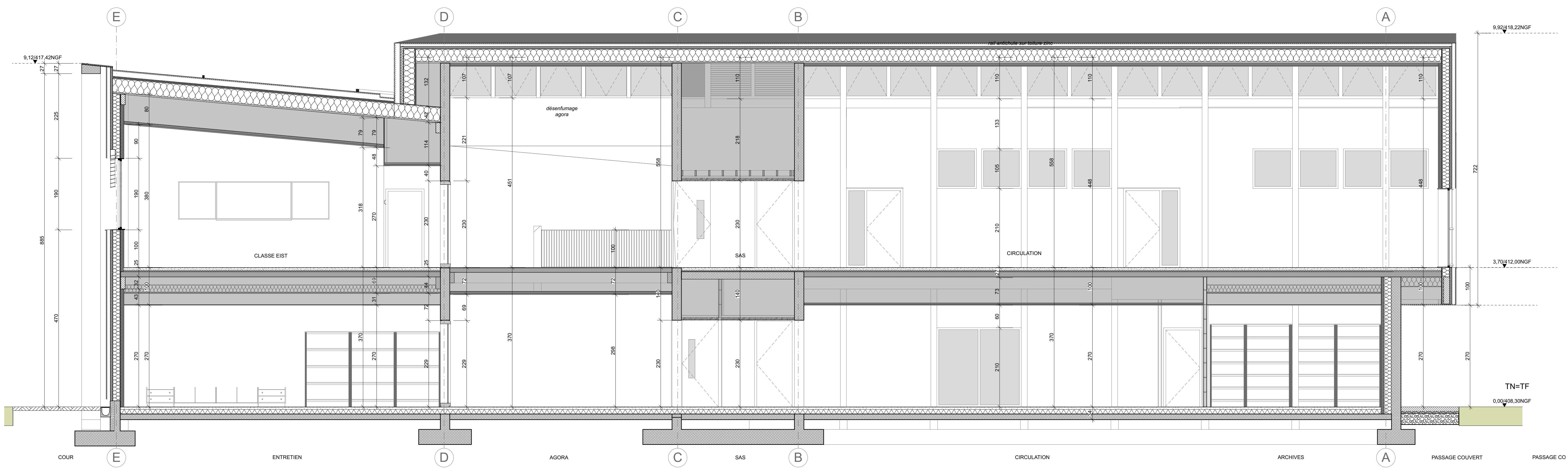
C - Coupe blocs 4/6 Nord
