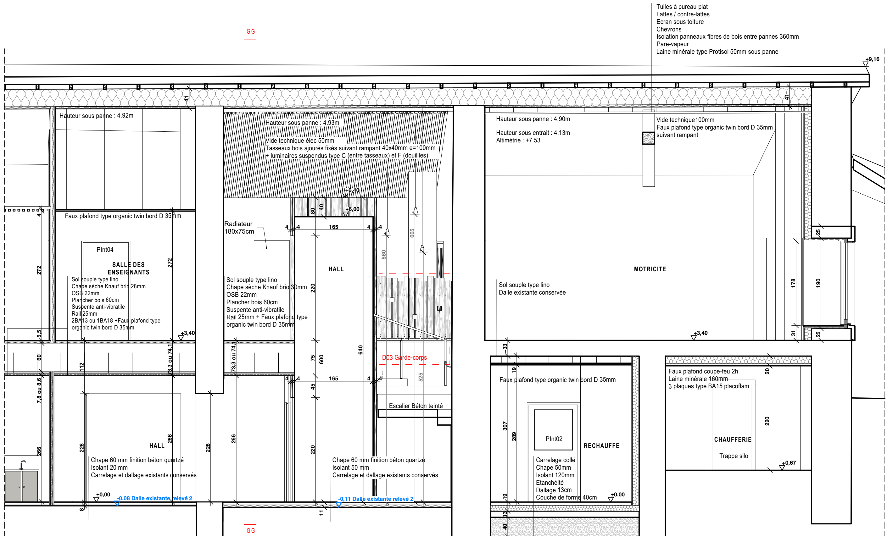
Coupe AA - Hall et motricité
