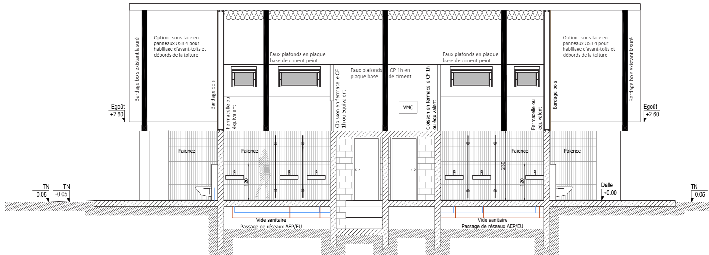
Coupe 02
