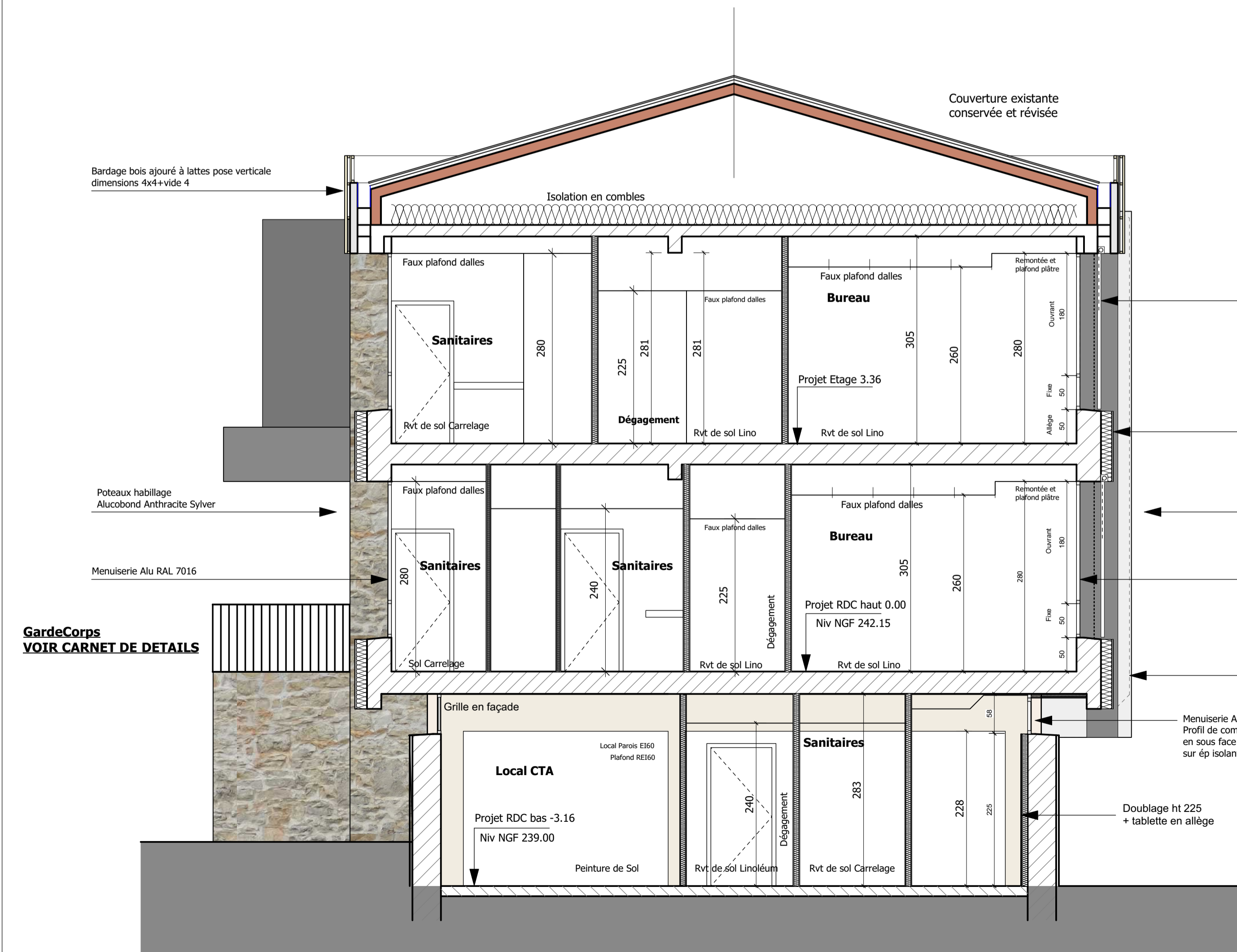
Coupe BB
