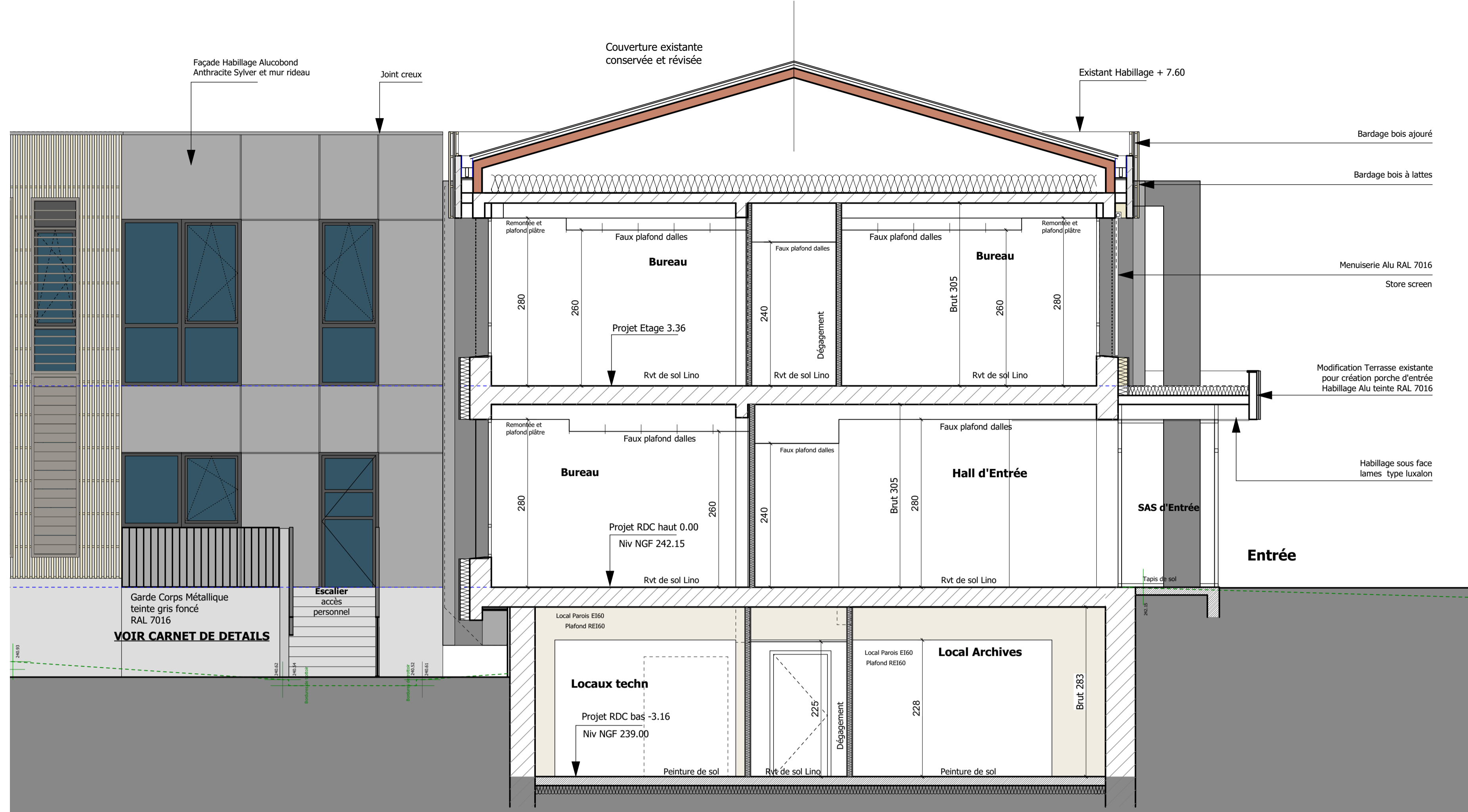
Coupe CC
