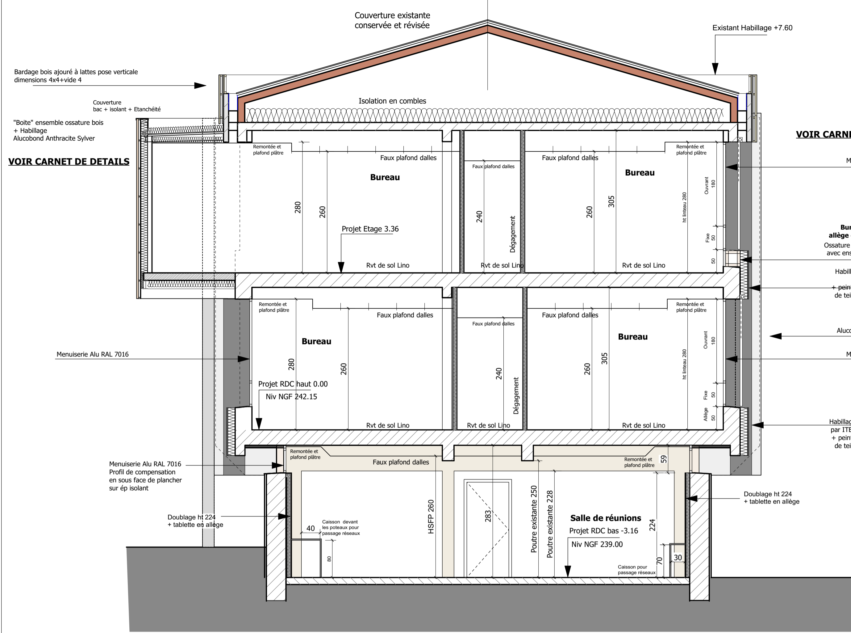
Coupe AA
