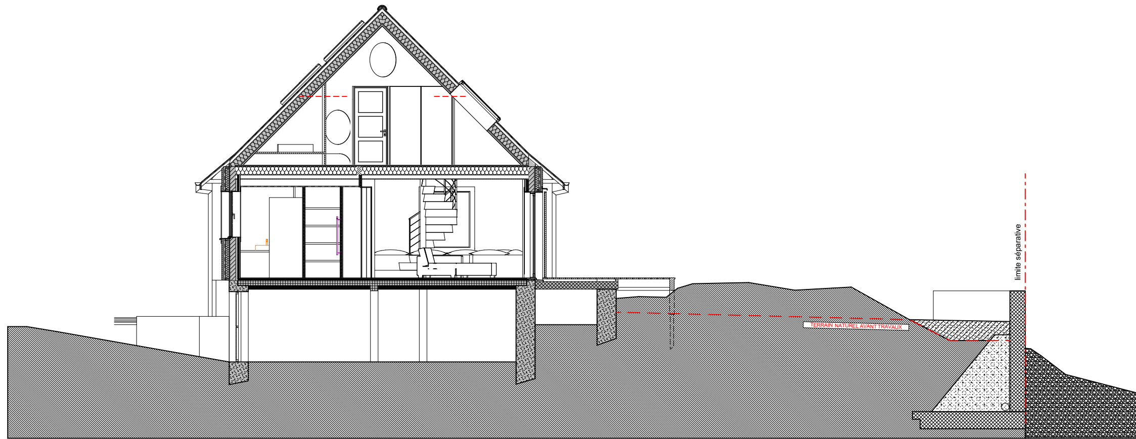
COUPE TRANSVERSALE BB' - Ech : 1/100
