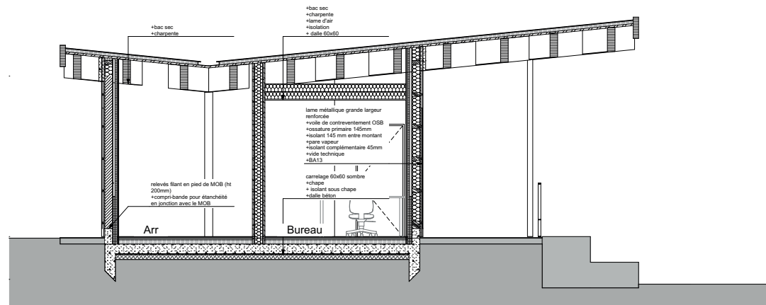
Coupe A éch:1/50°
