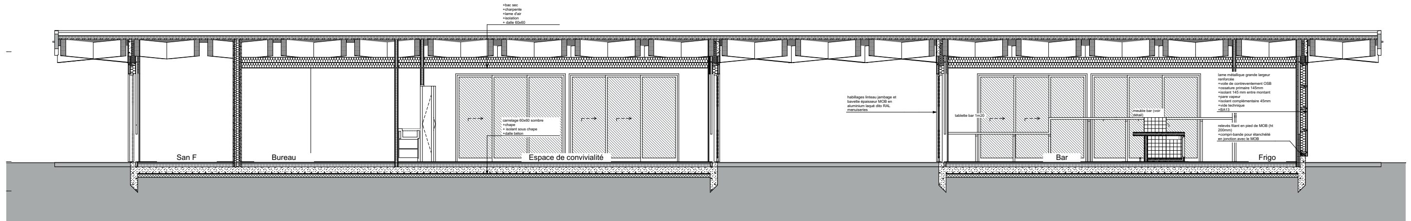
Coupe A éch:1/50°
