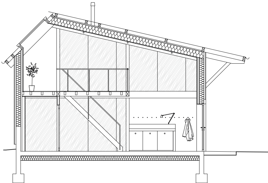
Coupe sur studio 1:100 e
