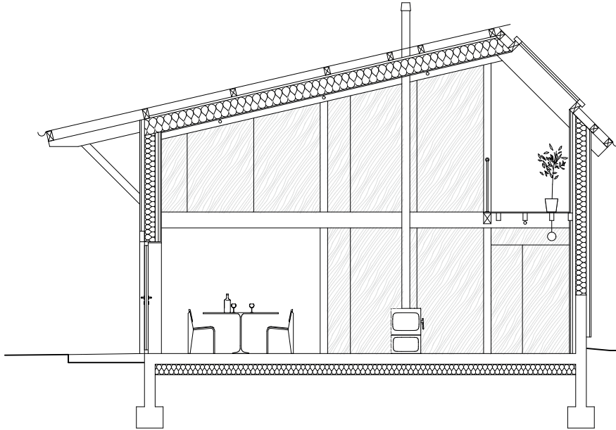
Coupe sur atelier de menuiserie 1:100 e
