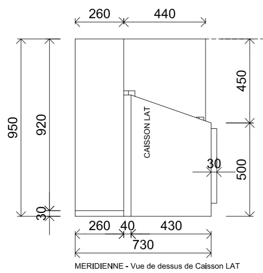
MERIDIENNE - Vue de dessus de Caisson LAT
