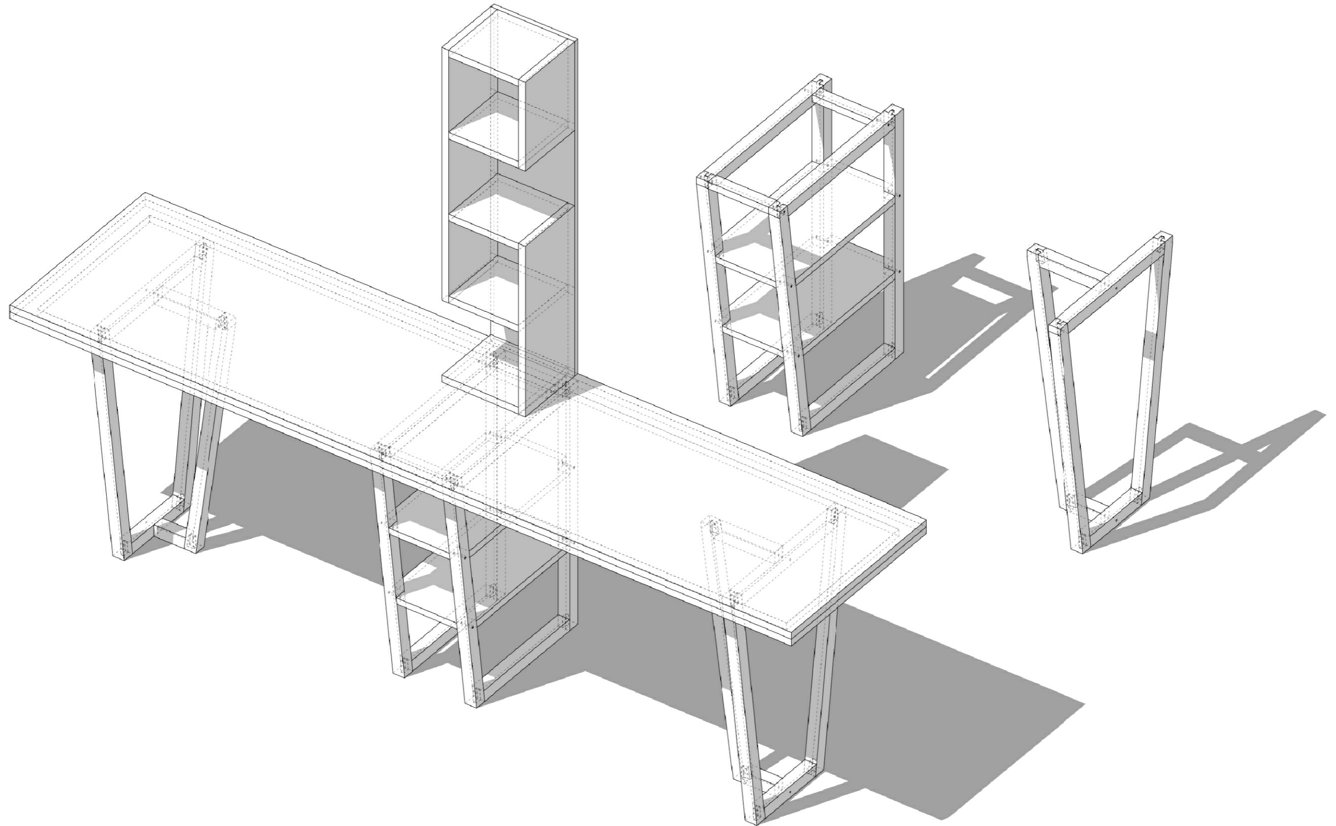
MANGE-DEBOUT Eclaté
