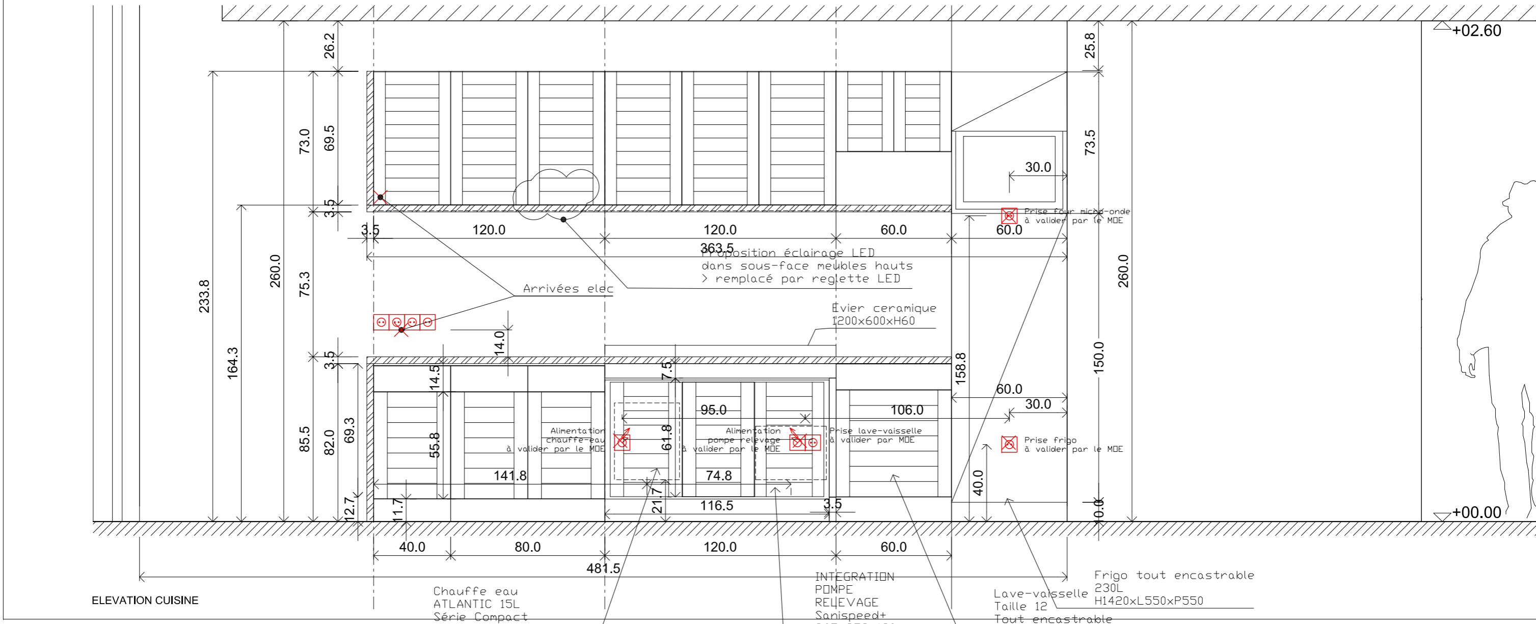
VUE CUISINE Dessin basé sur des éléments disponibles sur le bon coin - 40cm+80cm+120cm+60cm / HSP 260cm
