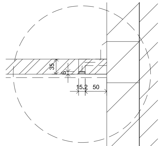
DETAIL SUR GOULOTTE LED - 1/5
