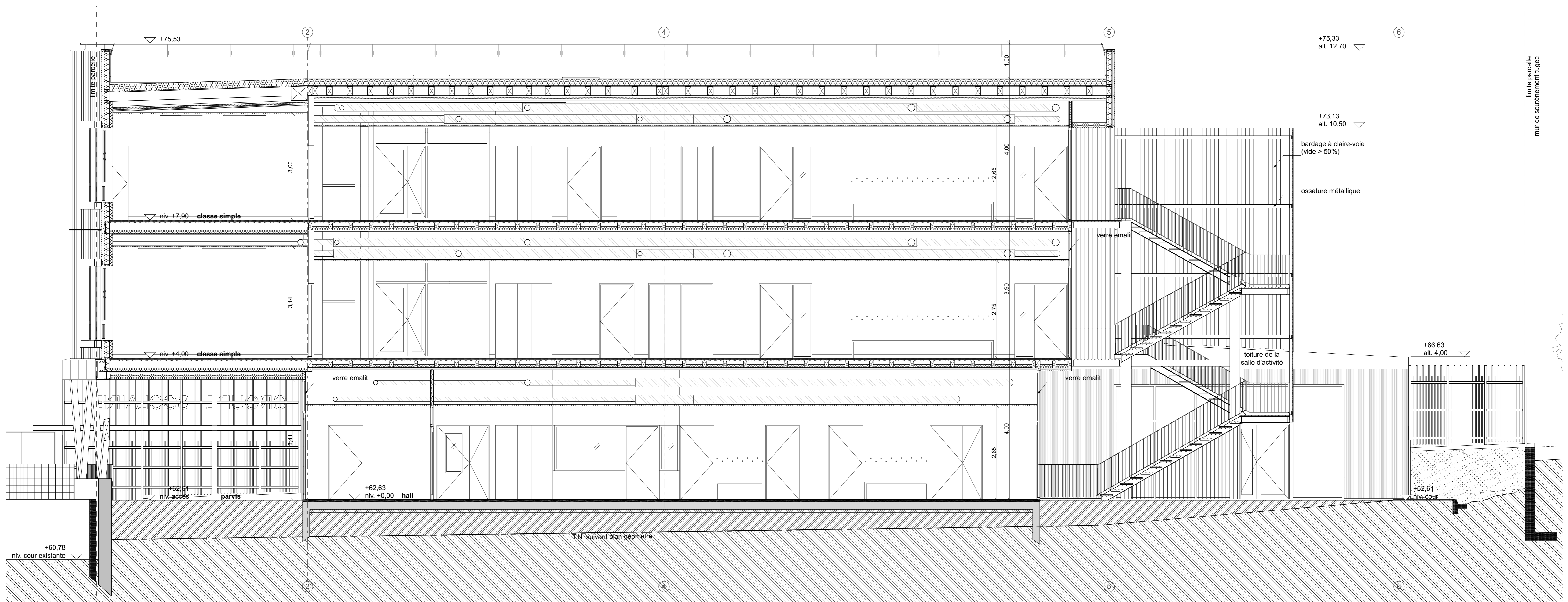
Coupe longitudinale D - dans la circulation
