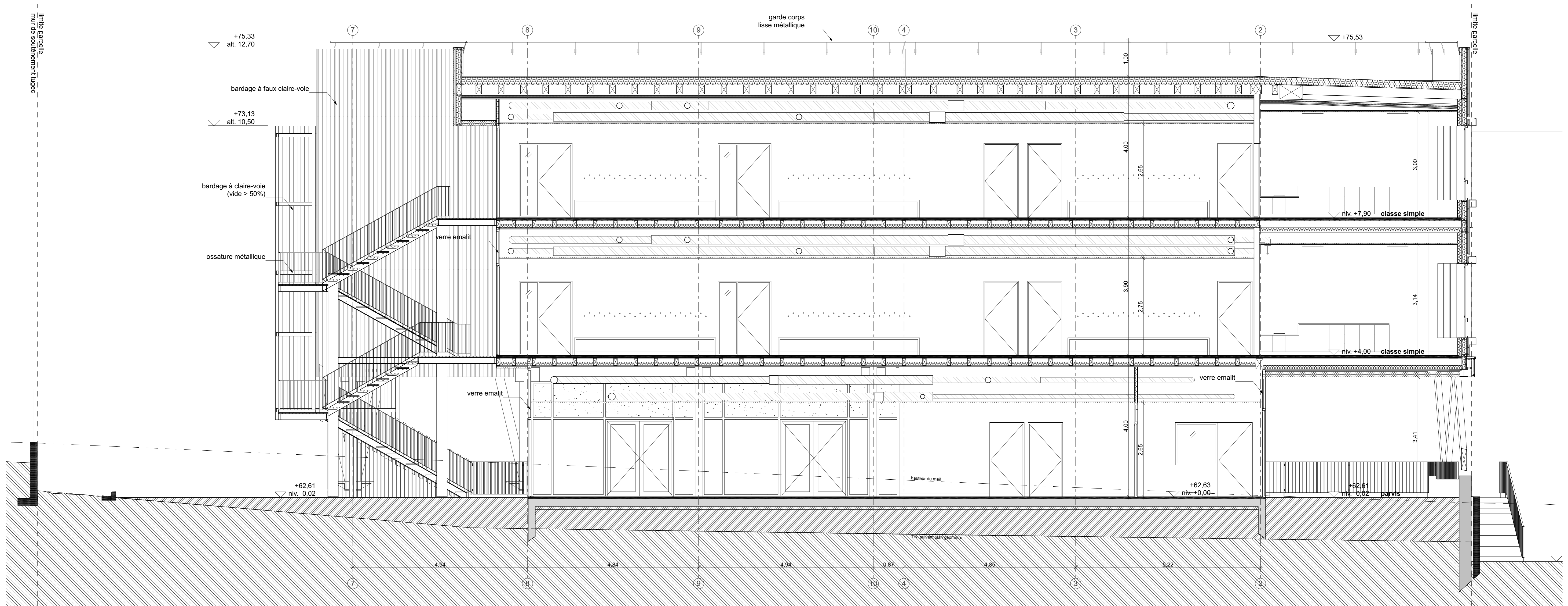
Coupe longitudinale A - dans la circulation
