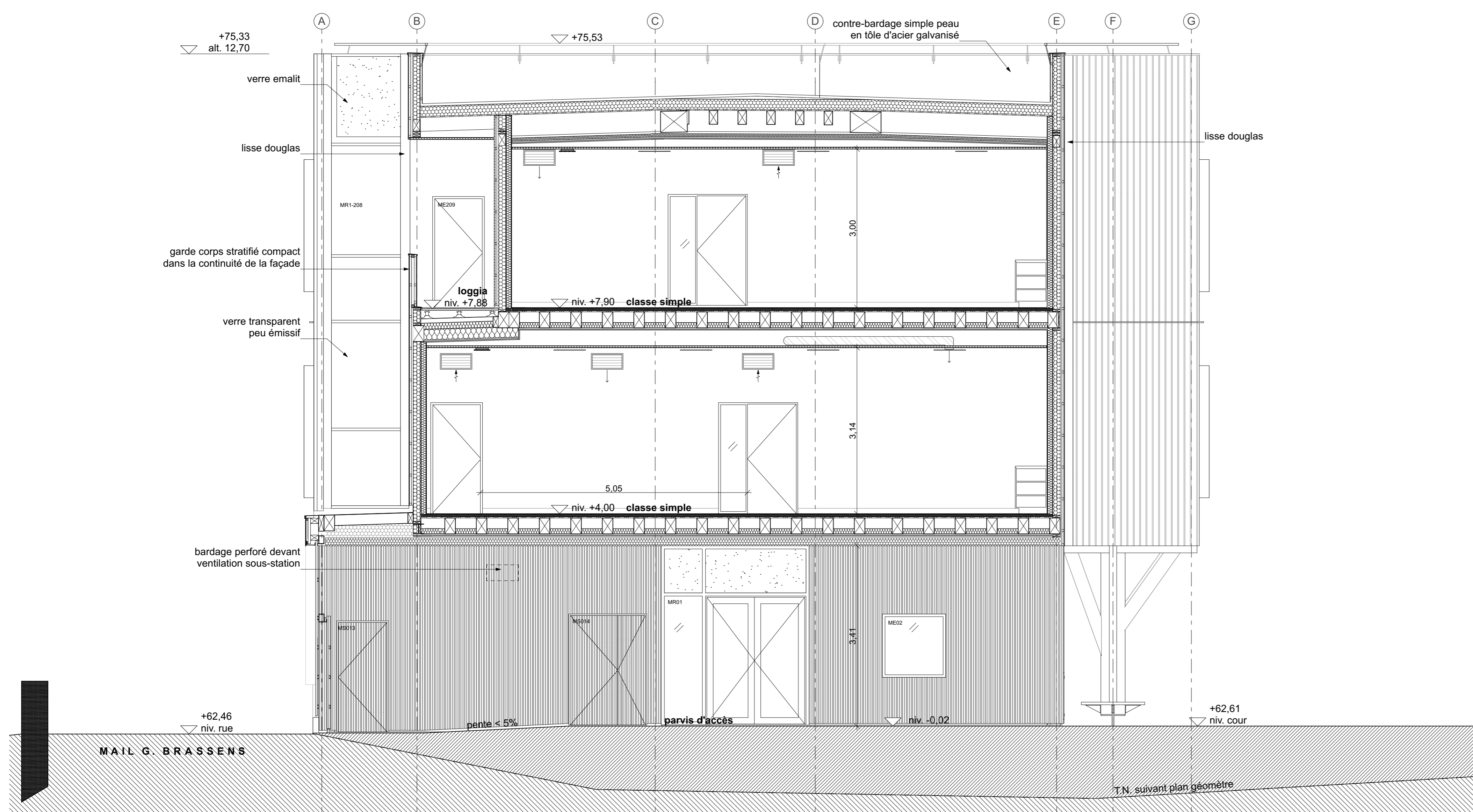
Coupe transversale E - dans le parvis d'accès
