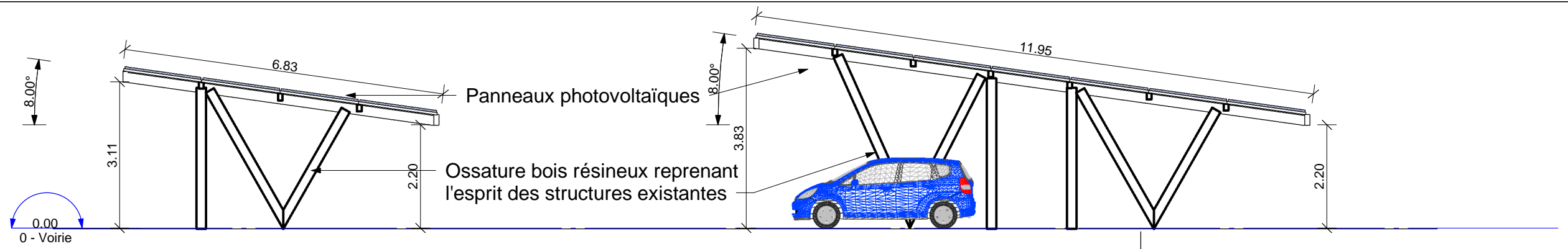
2 Coupe PC3 1 : 100
