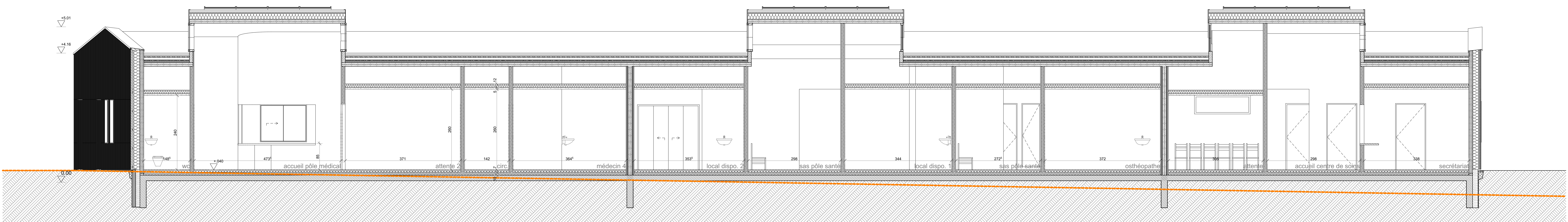
coupe L1
