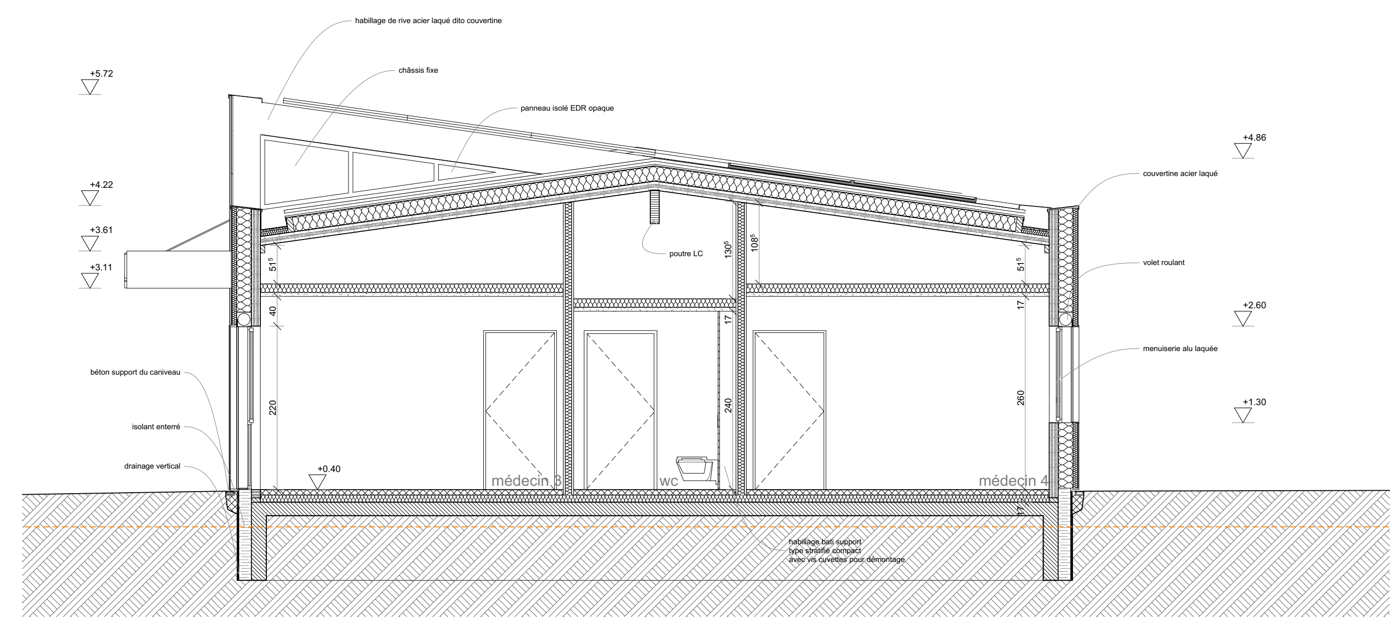
coupe T1
