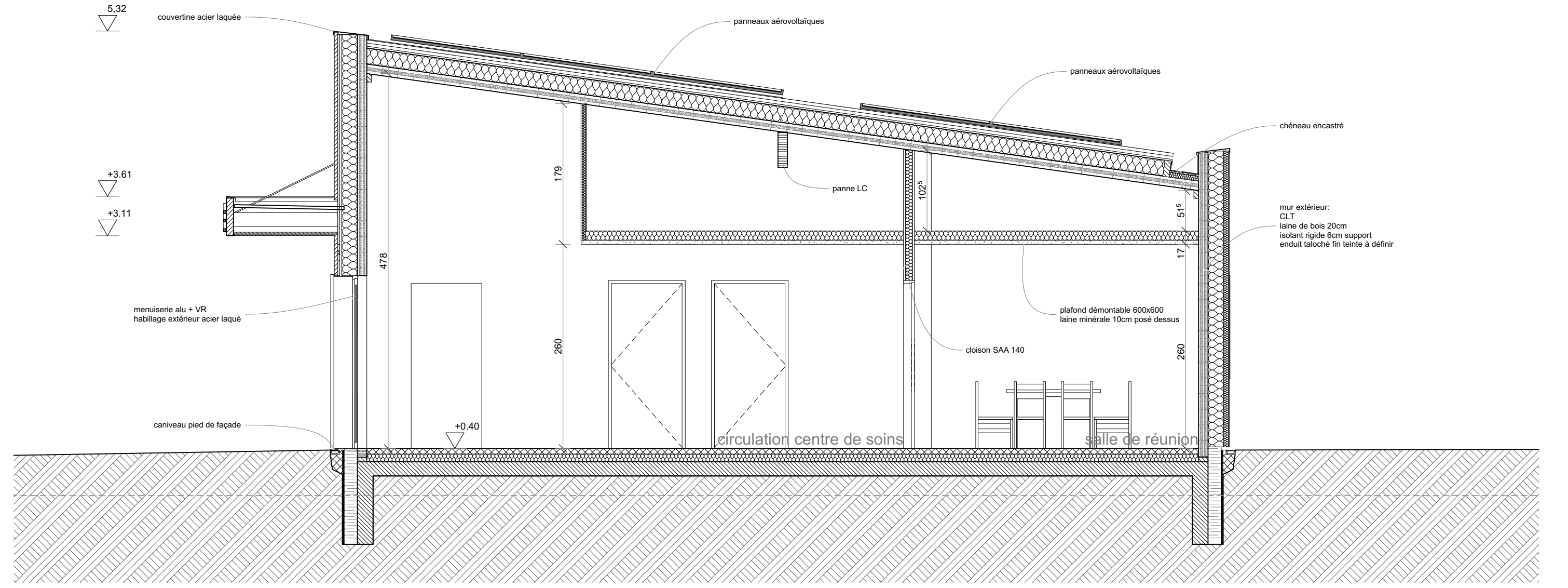
coupe T2
