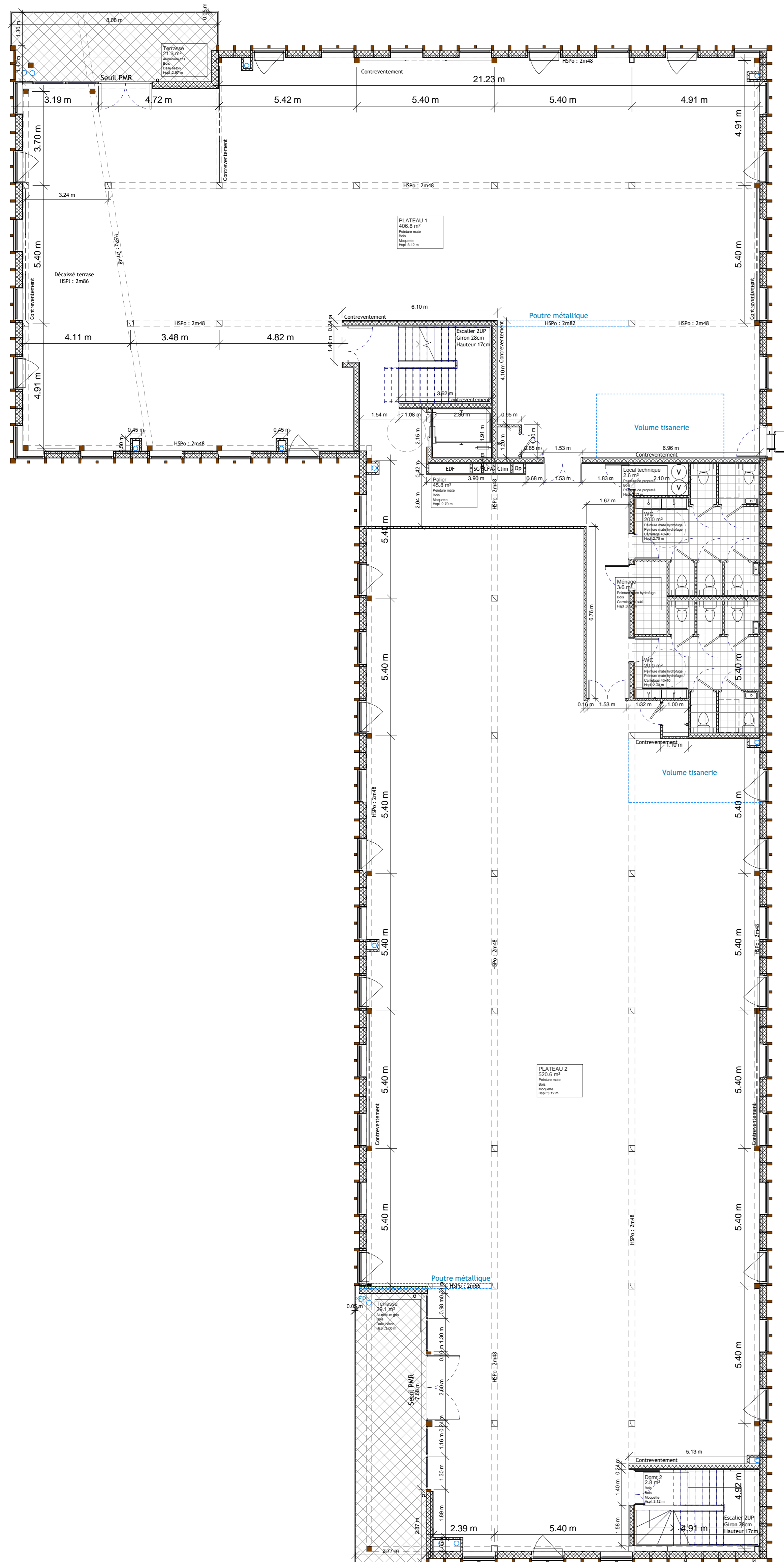
1 DCE 7 - NIVEAU R+1 1 : 100
